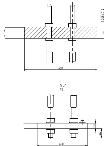
Fig. 4 Sezione verticale
