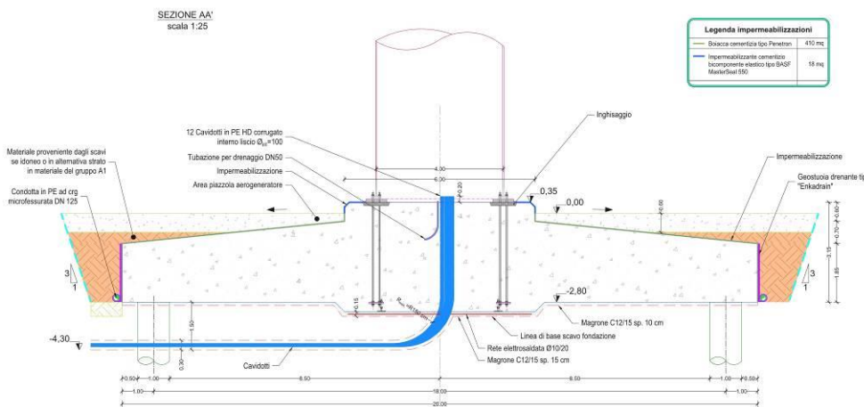
Fig. 2 Sezione del plinto
