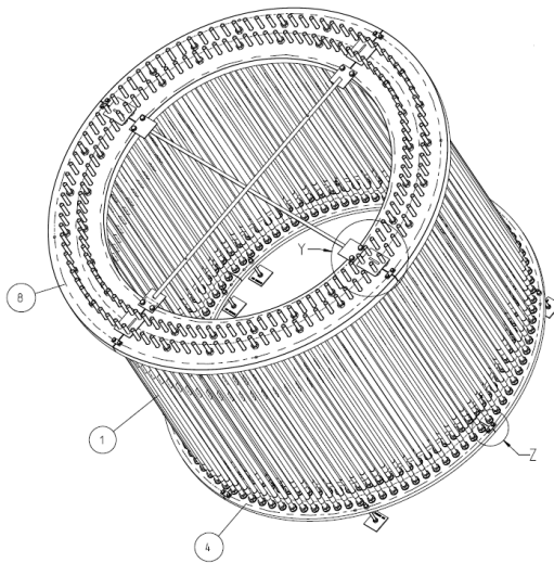
Fig. 3 Vista isometrica d'insieme
