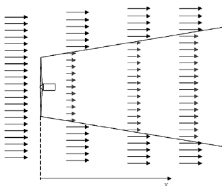
Figura 10 Andamento della scia provocata dalla presenza di un aerogeneratore. [Caffarelli-De Simone Principi di progettazione di impianti eolici Maggioli Editore]
