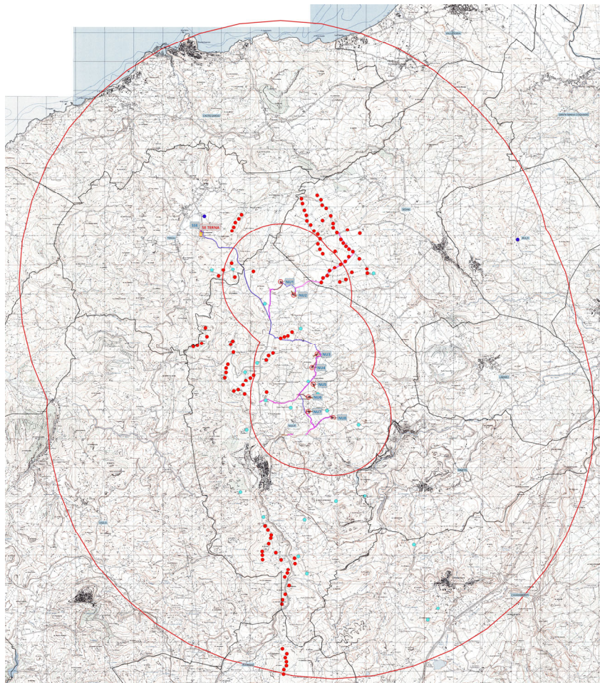
Figura 11 Impianti eolici presenti nel buffer di 9Km
