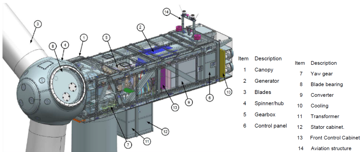
Figura 5 – Componenti dell'aerogeneratore
