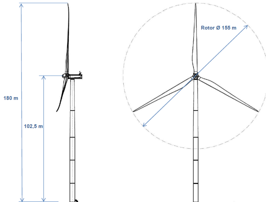
Figura 4 Schema geometrico degli aerogeneratori in progetto SG 6.0 - 155
