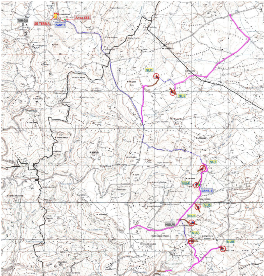
Figura 1 Layout progetto definitivo su base IGM
