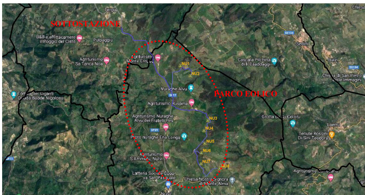
Figura 3 – Vista satellitare del posizionamento del parco eolico “Mattesuija” in progetto
