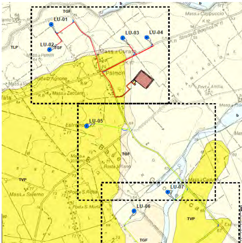
Inquadramento geologico di dettaglio
