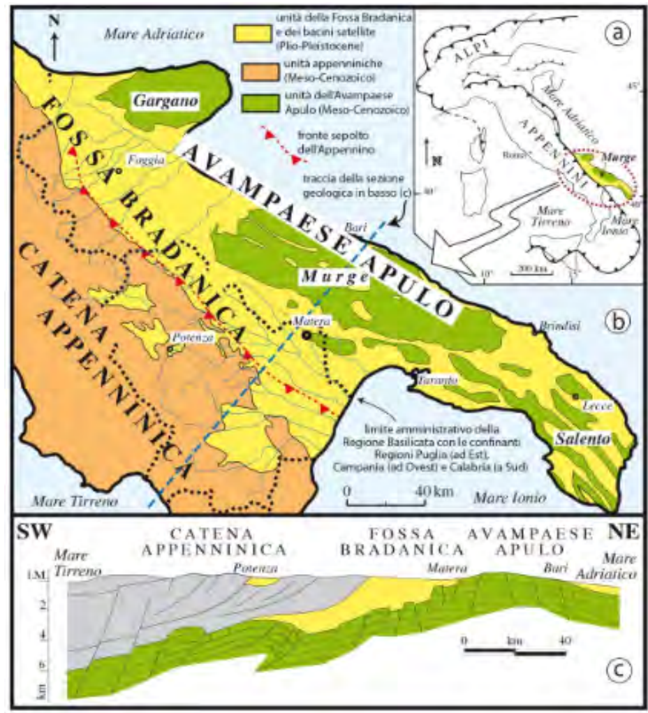
Schema Tettonico
