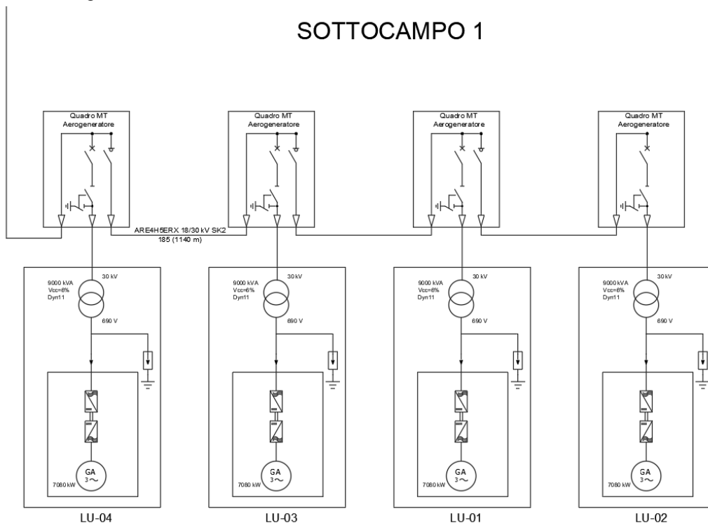
Schema a blocchi del parco eolico GRUPPO 1
