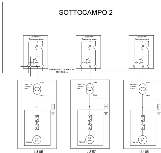
Schema a blocchi del parco eolico GRUPPO 2
