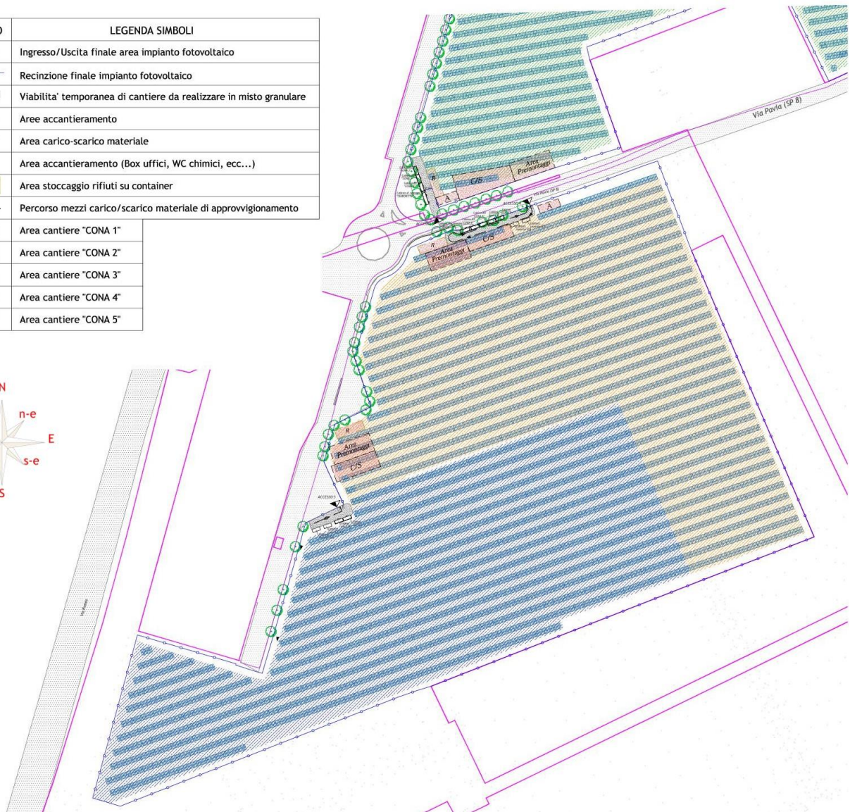
Figura 9 - Aree di cantiere impianti "CONA 4" e "CONA 5"
