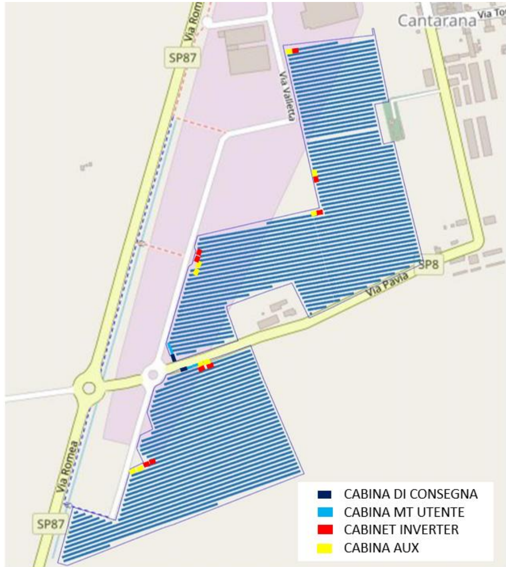
Figura 2 - Vista planimetrica stato futuro
