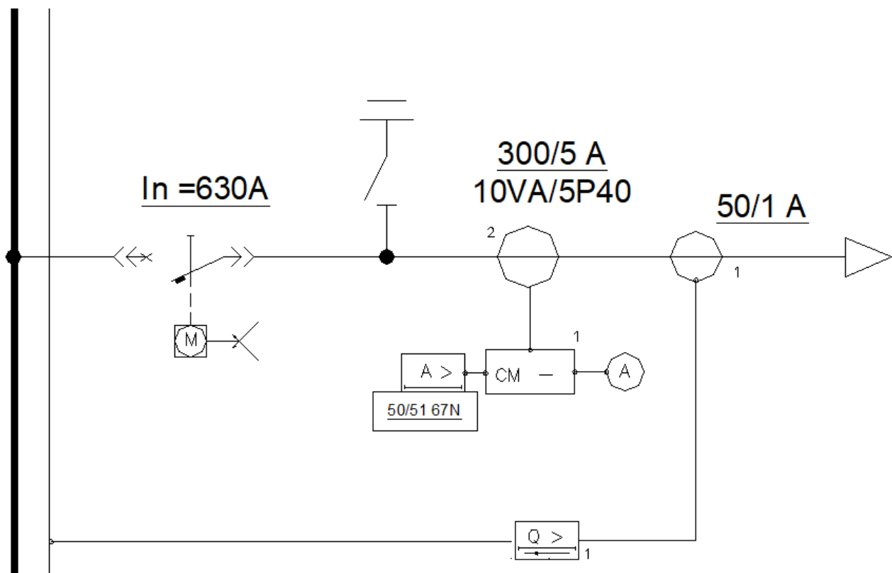
Particolare di un quadro 36 kV scomparto linea
