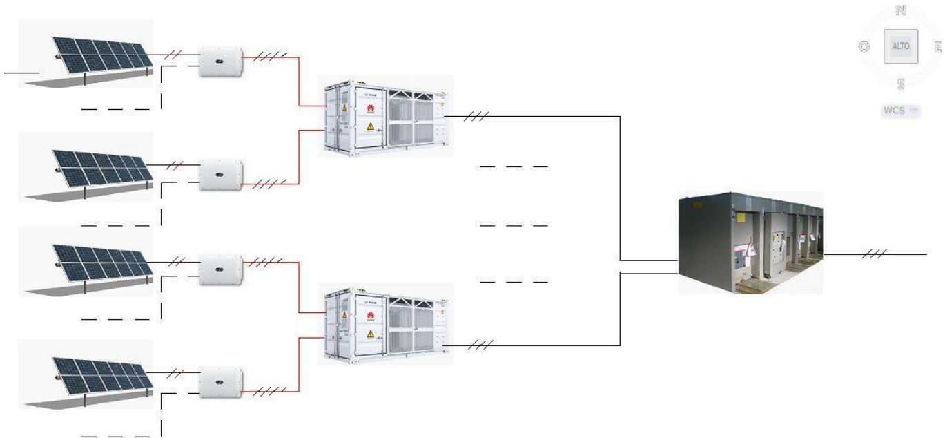
Schema di principio della linea di produzione elettrica (moduli-inverter-trasformazione-immissione in rete)
