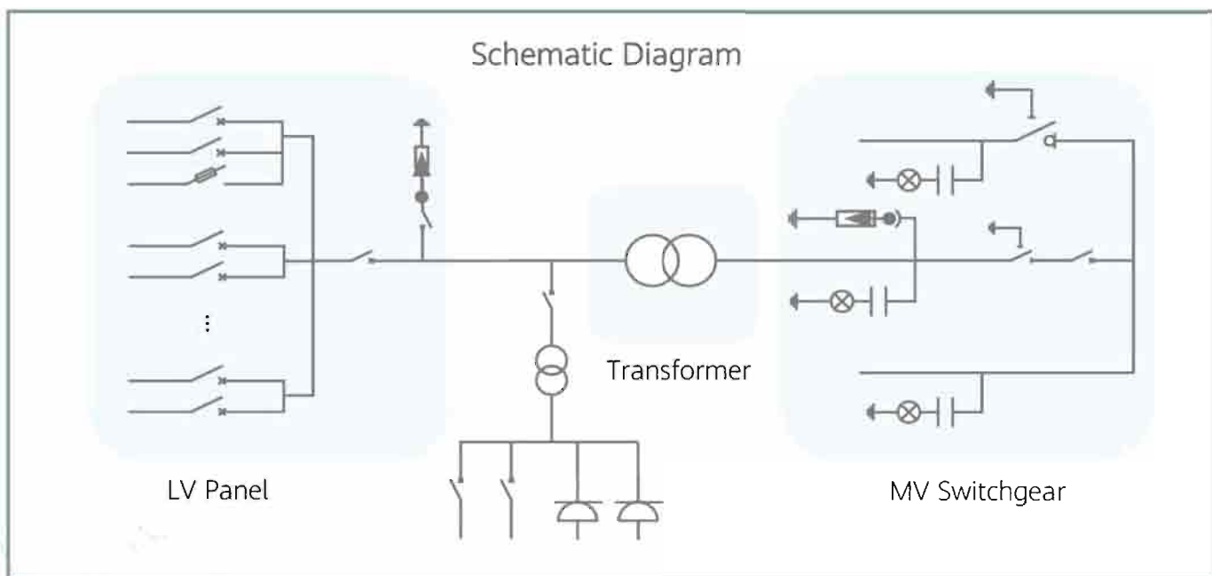
schema unifilare di principio della UP
