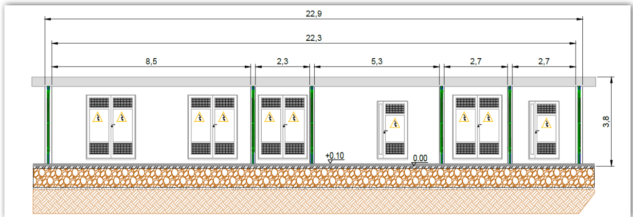
Prospetto principale dei locali tecnici della SSE.
