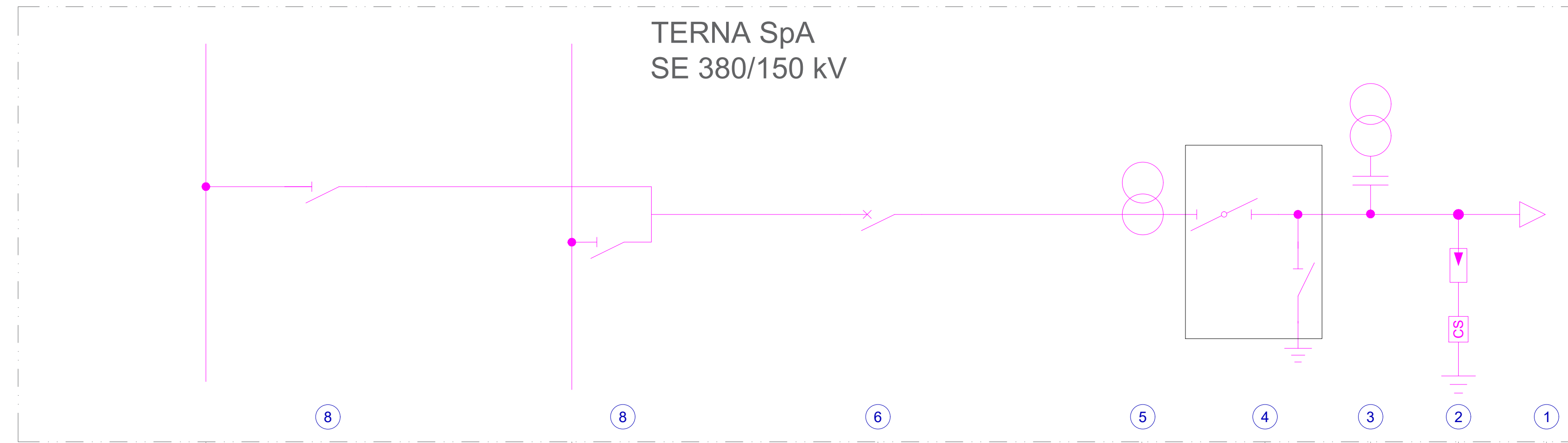
Pianta, profilo elettromeccanico e schema unifilare Stallo di Consegna AT in area TERNA - scala 1:100
