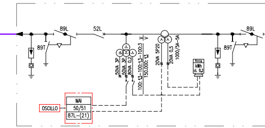
Stallo Partenza linea AT 150 kV per la condivisione di stallo
