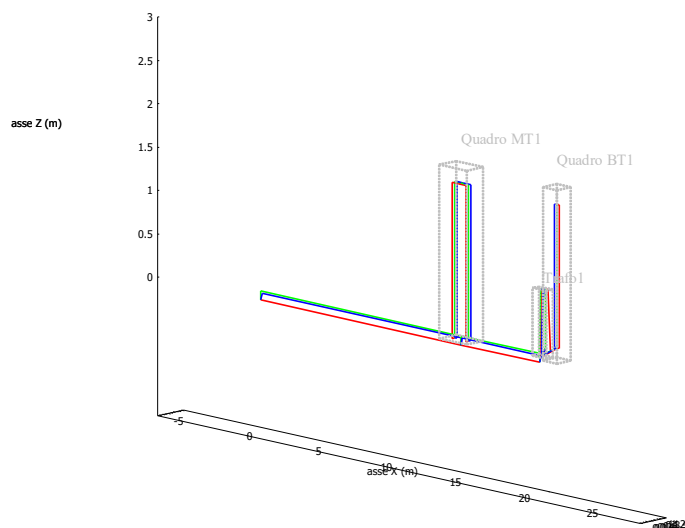
Fig.8 - Modello spaziale cablaggi nella cabina di ricezione
