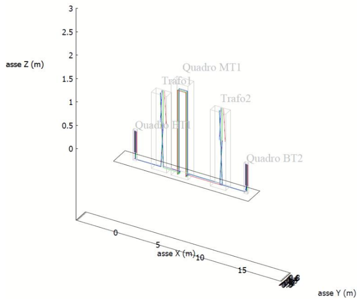
Fig.7 - Modello spaziale cablaggi nelle cabine di trasformazione MT/BT da 4.000 kVA
