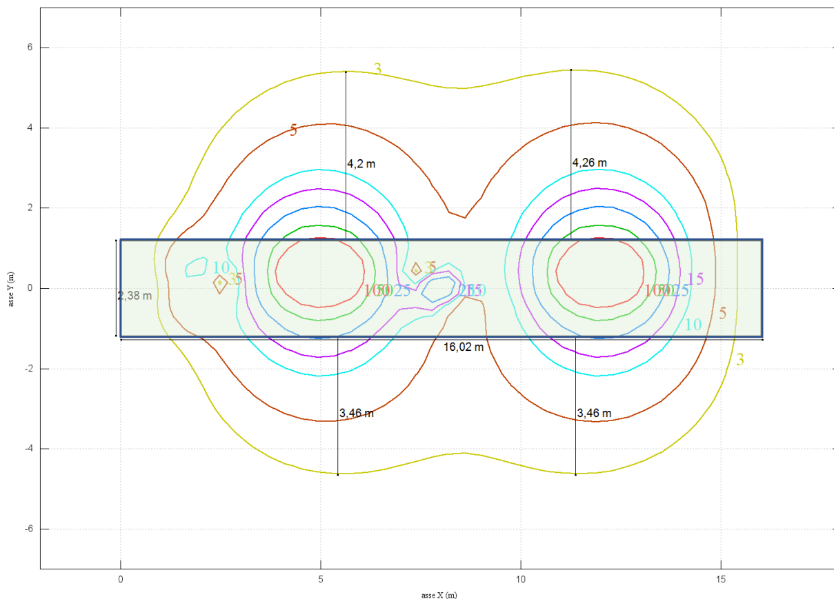
Cabina - calcolo su piano xy - quote Z=1,33 m
