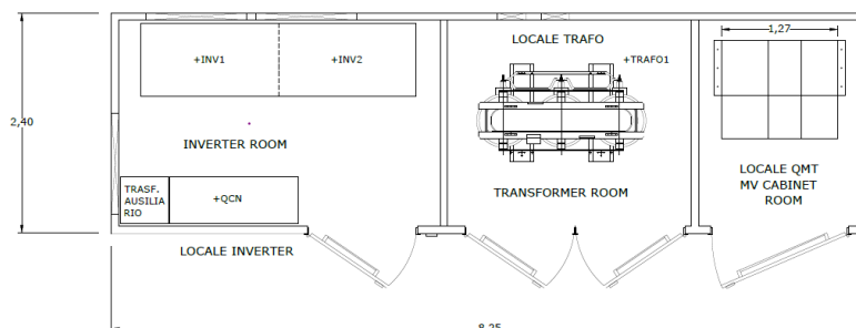
Fig.4 - Ingombri cabine di trasformazione MT/BT da 2.000 kVA
