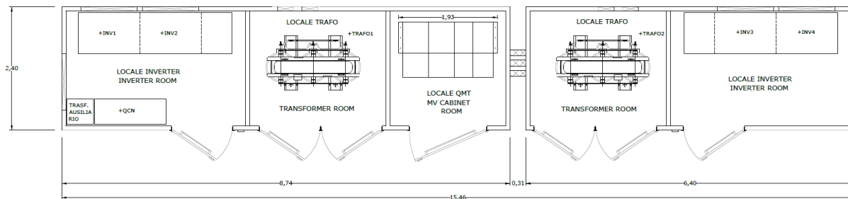
Fig.5 - Ingombri cabine di trasformazione MT/BT da 4.000 kVA
