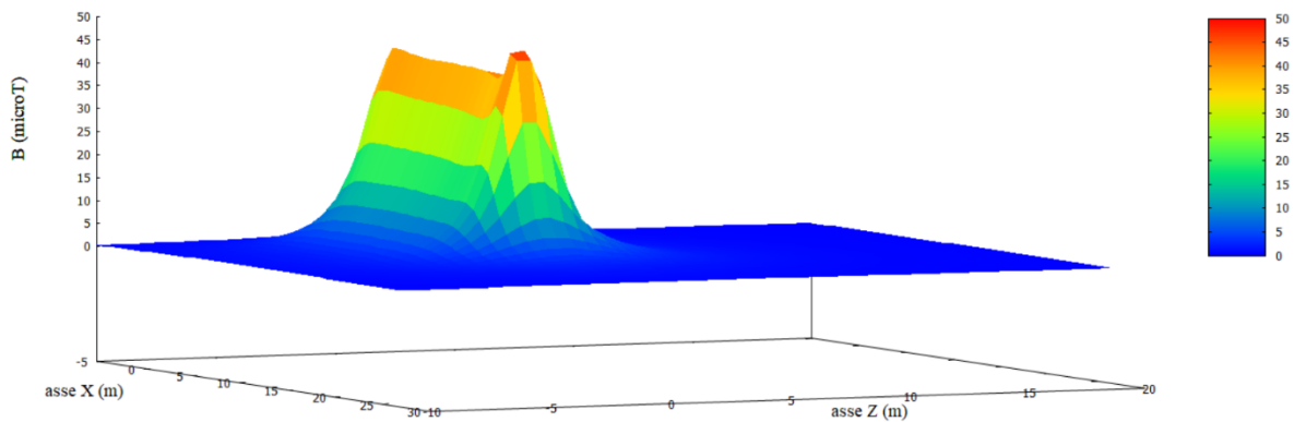
Cabina - calcolo su piano xz - quote Y=-1 m
