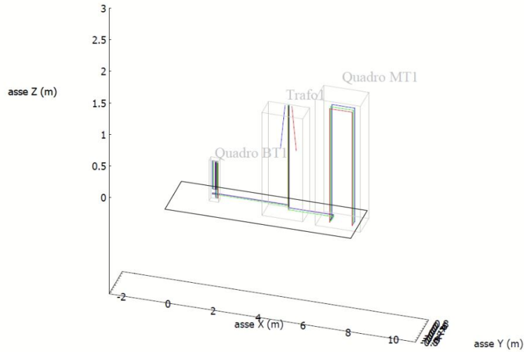
Fig.7 - Modello spaziale cablaggi nelle cabine di trasformazione MT/BT da 2.000 kVA
