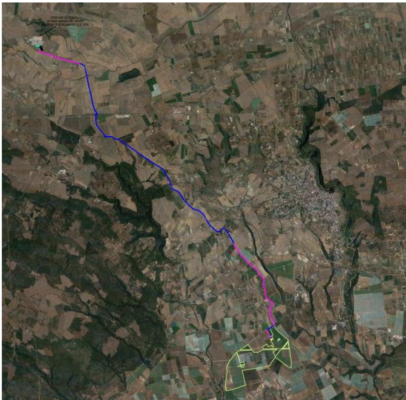
Fig. 2 – Ortofoto dell’area oggetto d’intervento e del tracciato del cavidotto fino alla SEU Utente condivisa
