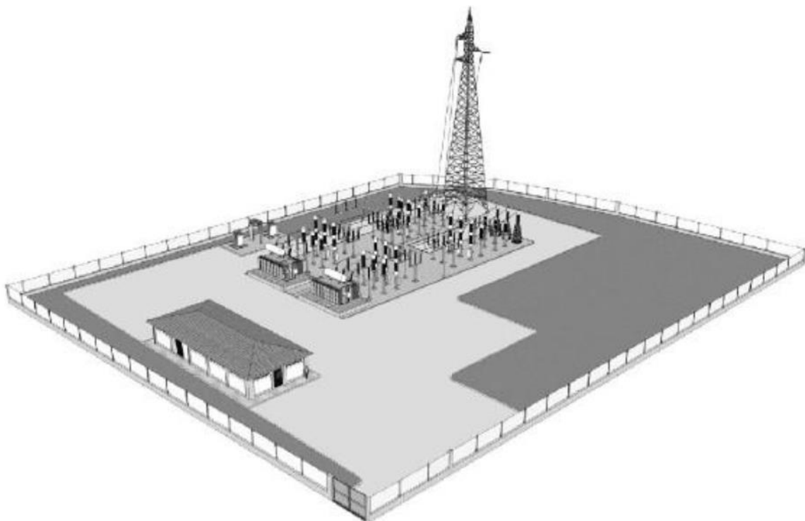
Fig. 3a: Rappresentazione di una tipica Stazione di Utensia 150/20 kV con apparecchiature isolate in aria
