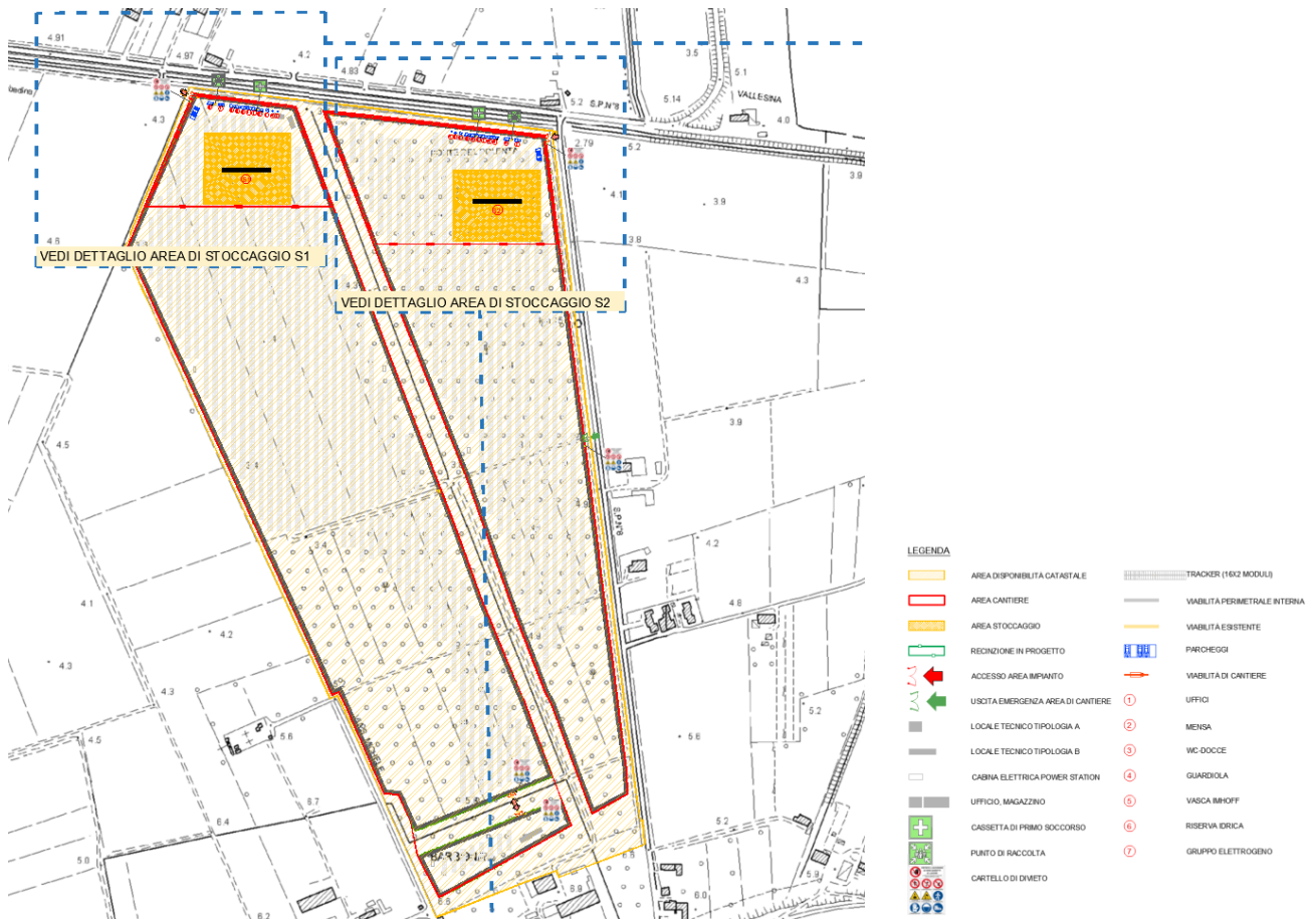
Figura 4.1: Planimetria di cantiere
