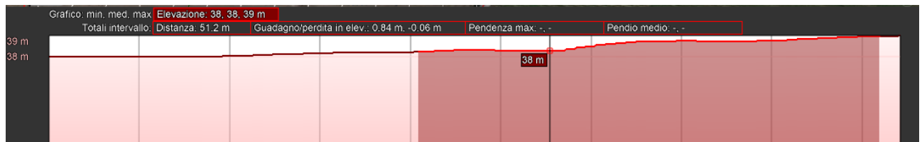
Figura 7-70 Sez. 65 in direzione nord sud sul sito di installazione FV-La Gonnella
