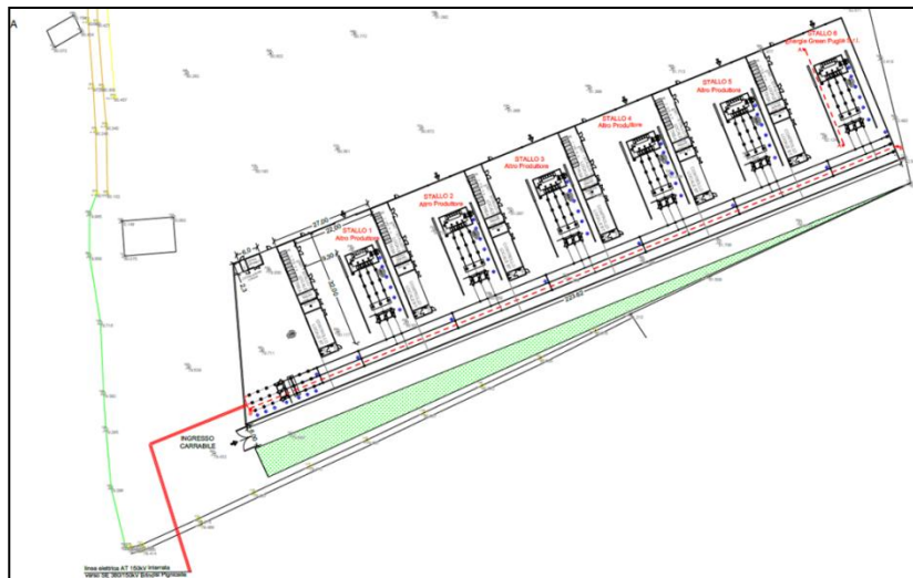
Figura 4-7 Planimetria Sottostazione Utente
