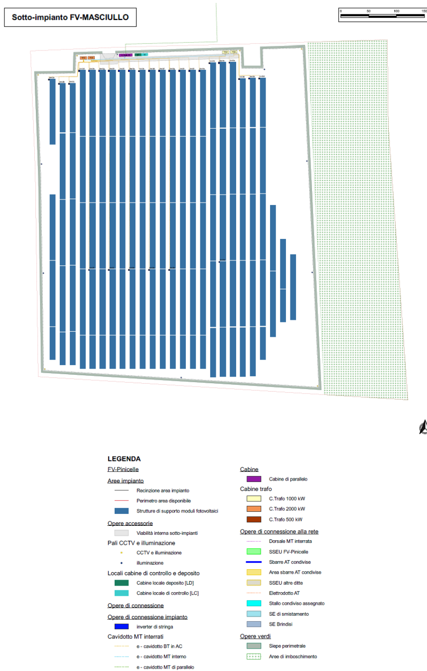
Figura 4-3 Layout delle opere di connessione elettrica interne al sotto-impianto "FV - Masciullo"
