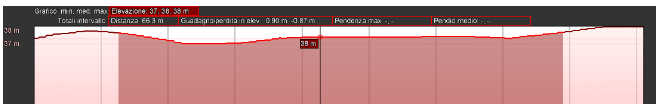
Figura 7-78 Sez. 73 in direzione nord sud sul sito di installazione FV-La Gonnella
