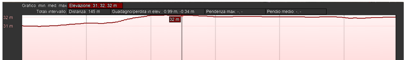
Figura 7-30 Sez. 28 in direzione nord sud sul sito di installazione FV-Casignano
