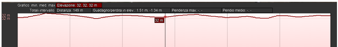
Figura 7-27 Sez. 25 in direzione nord sud sul sito di installazione FV-Casignano
