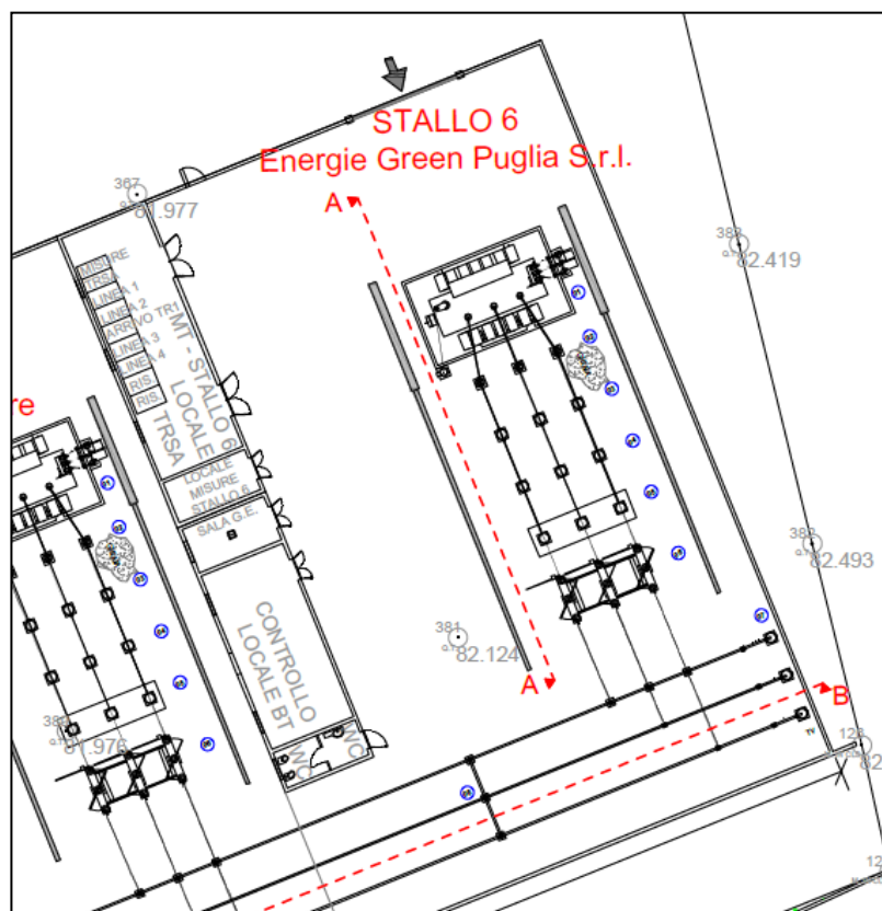
Figura 4-8 Dettaglio - Stallo 6 Energie Green Puglia srl
