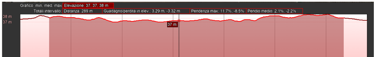
Figura 7-47 Sez. 43 in direzione nord sud sul sito di installazione FV-Masciullo
