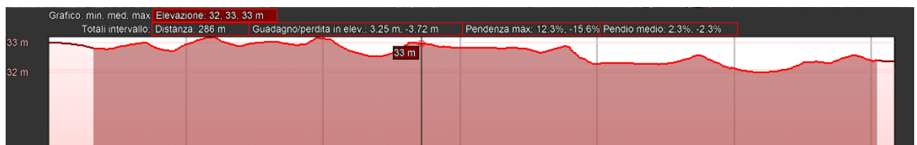
Figura 7-14 Sez. 12 in direzione nord sud sul sito di installazione FV-Casignano
