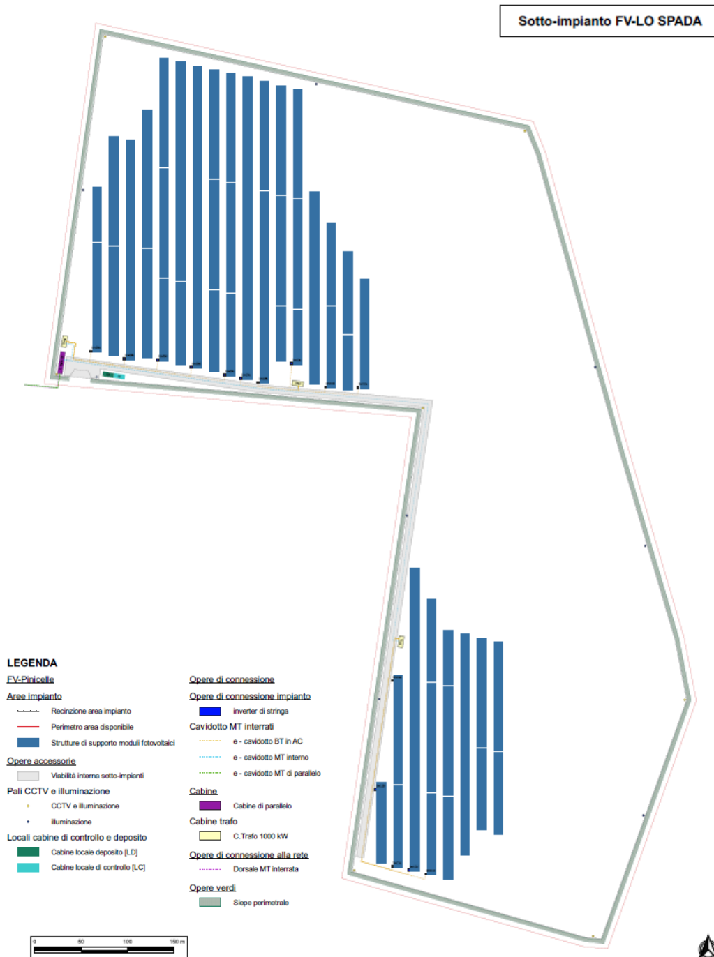
Figura 4-4 Layout delle opere di connessione elettrica interne al sotto-impianto “FV - Lo Spada”
