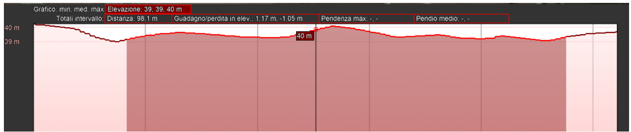
Figura 7-62 Sez. 57 in direzione nord sud sul sito di installazione FV-La Gonnella
