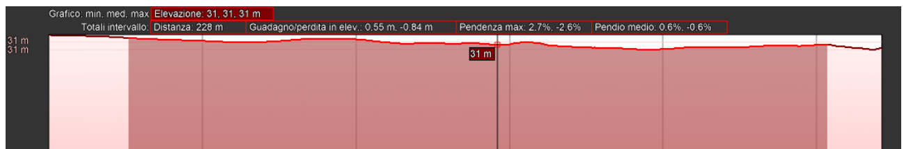
Figura 7-20 Sez. 18 in direzione nord sud sul sito di installazione FV-Casignano
