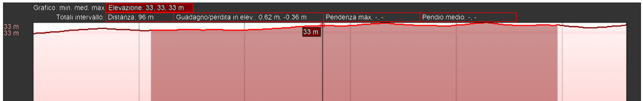
Figura 7-25 Sez. 23 in direzione nord sud sul sito di installazione FV-Casignano
