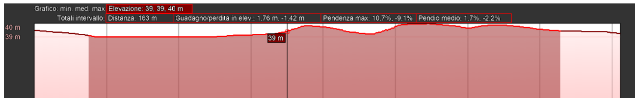
Figura 7-64 Sez. 59 in direzione nord sud sul sito di installazione FV-La Gonnella
