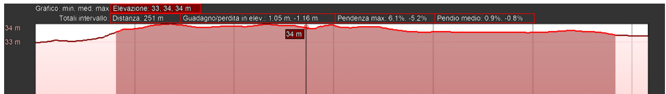
Figura 7-11 Sez. 9 in direzione nord sud sul sito di installazione FV-Casignano
