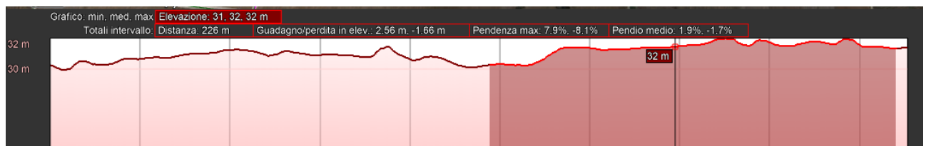
Figura 7-41 Sez. 38 in direzione nord sud sul sito di installazione FV-Lo Spada
