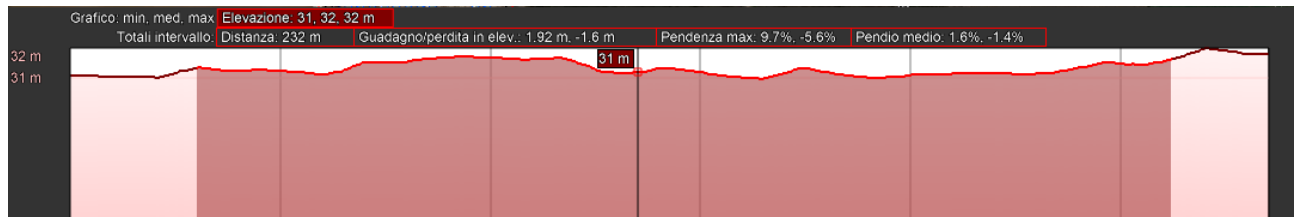
Figura 7-18 Sez. 16 in direzione nord sud sul sito di installazione FV-Casignano
