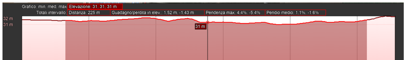
Figura 7-19 Sez. 17 in direzione nord sud sul sito di installazione FV-Casignano
