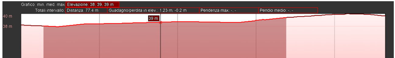
Figura 7-68 Sez. 63 in direzione nord sud sul sito di installazione FV-La Gonnella
