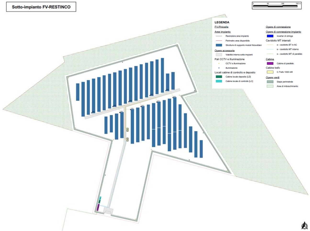
Figura 4-5 Layout delle opere di connessione elettrica interne al sotto-impianto "FV - Restinco"
