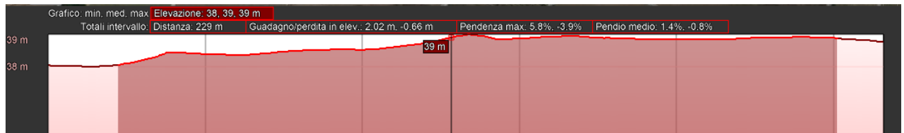
Figura 7-63 Sez. 58 in direzione nord sud sul sito di installazione FV-La Gonnella
