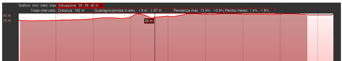
Figura 7-66 Sez. 61 in direzione nord sud sul sito di installazione FV-La Gonnella
