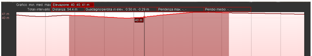
Figura 7-56 Sez. 51 in direzione nord sud sul sito di installazione FV-La Gonnella
