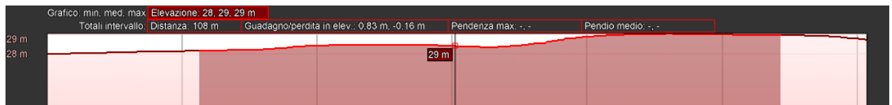
Figura 7-3 Sez. 2 in direzione nord sud sul sito di installazione FV-Restinco
