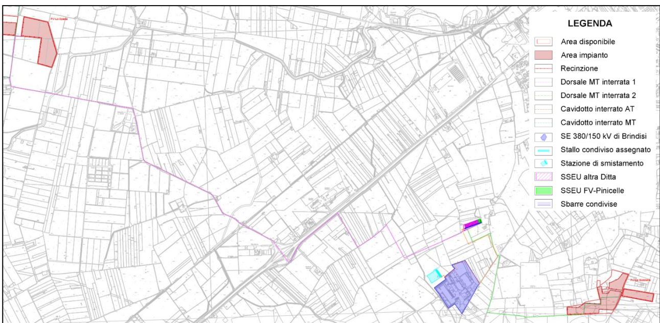
Figura 4-1 Schema di convogliamento dell'energia dalle cabine di parallelo ubicate rispettivamente nei sotto-impianti FV-La Gonnella e FV-Lo Spada alla Sottostazione Elettrica Utente 150/30 kV (SSEU FV-Pinicelle) e da questa allo stallo condiviso assegnato, da realizzare in una futura stazione di smistamento 150 kV da costruire nelle immediate vicinanze della Stazione di Trasformazione 380/150 kV "Brindisi"
