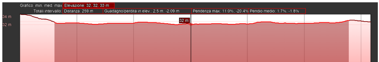
Figura 7-16 Sez. 14 in direzione nord sud sul sito di installazione FV-Casignano
