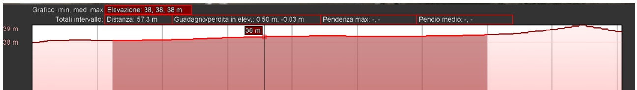
Figura 7-75 Sez. 70 in direzione nord sud sul sito di installazione FV-La Gonnella
