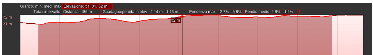
Figura 7-37 Sez. 34 in direzione nord sud sul sito di installazione FV-Lo Spada
