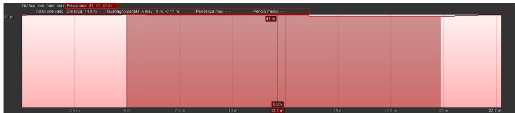
Figura 8-6 Sez. 82 in direzione nord sud sul sito nel quale verrà realizzata la SSEU FV-Pinicelle
