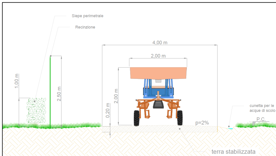
Figura 6-9 Dettaglio costruttivo delle strade per la viabilità interna al sito di installazione dell'impianto fotovoltaico
