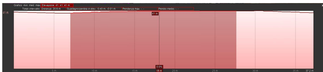
Figura 8-2 Sez. 78 in direzione nord sud sul sito nel quale verrà realizzata la SSEU FV-Pinicelle
