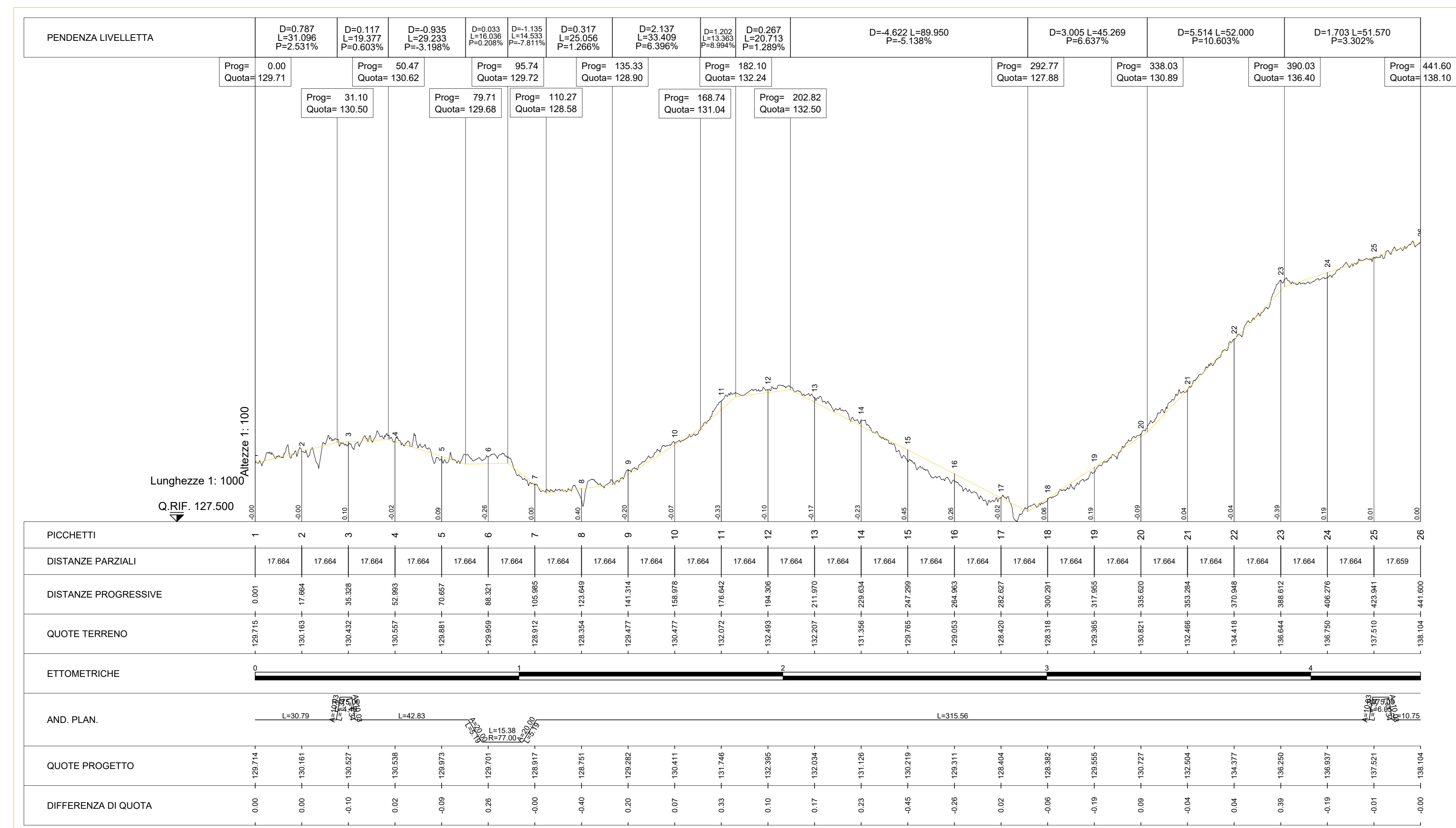
SEZIONE ASSE STRADA_4 - TRATTO FF' _scala 1:100
