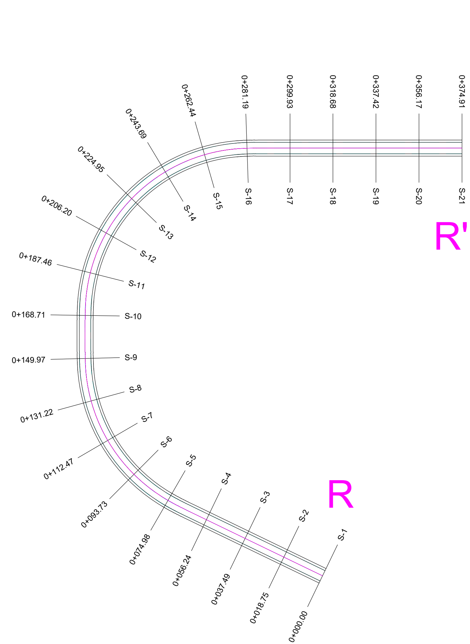
PLANIMETRIA STRADA_12 - TRATTO RR' _ scala 1:1000
