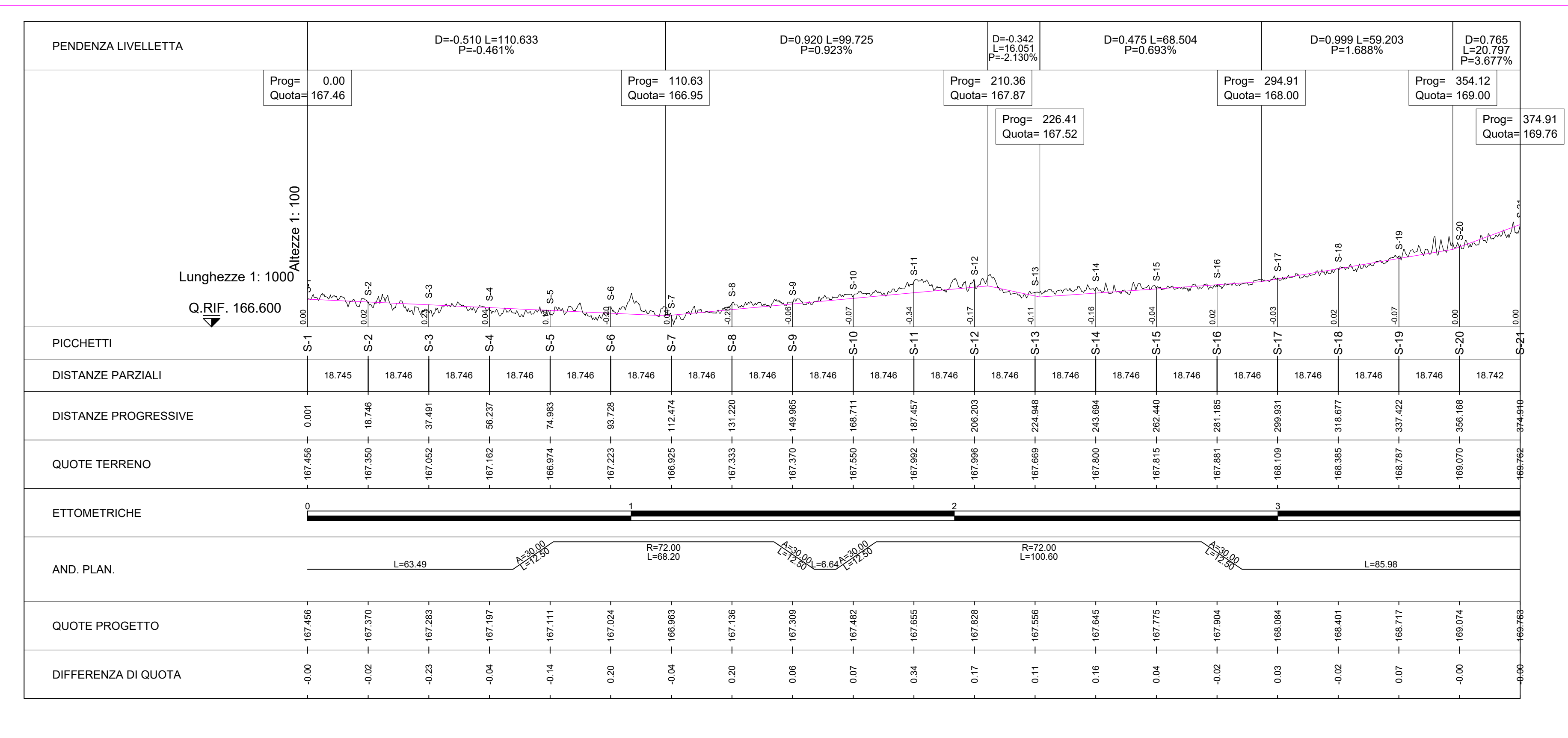
SEZIONE ASSE STRADA_12 - TRATTO RR' _ scala 1:100
