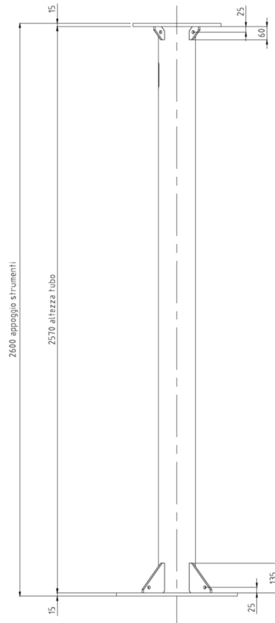
Fig. 3 – Sostegno TA
