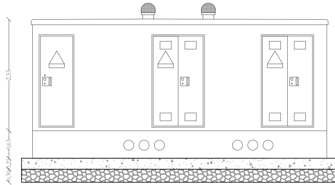
Prospetto Sud
