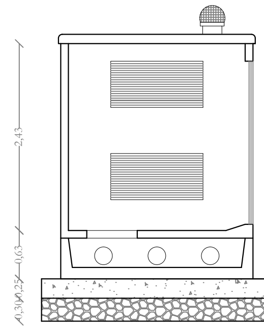
Sezione A-A
