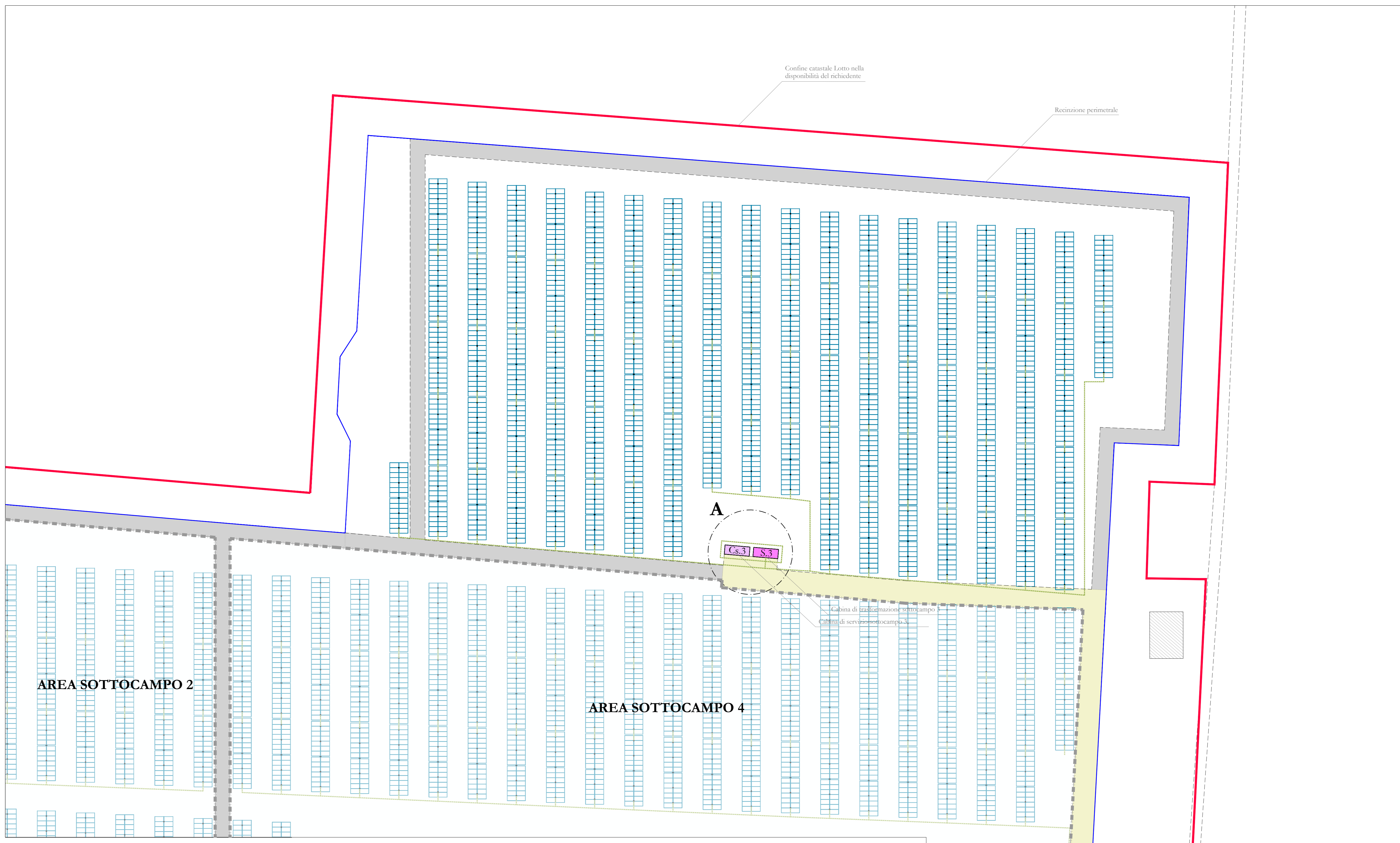
Planimetria generale con indicazione delle sezioni elettriche "AREA 1" - scala 1:2.000
