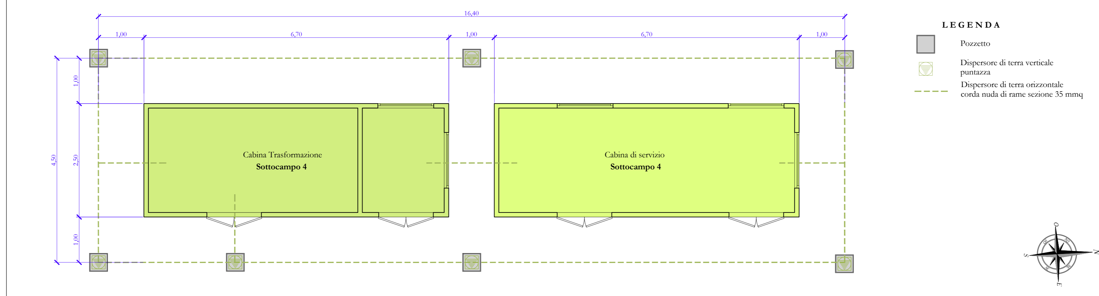
Planimetria impianto di terra, Sottocampo 4 "AREA 1" - scala 1:500
