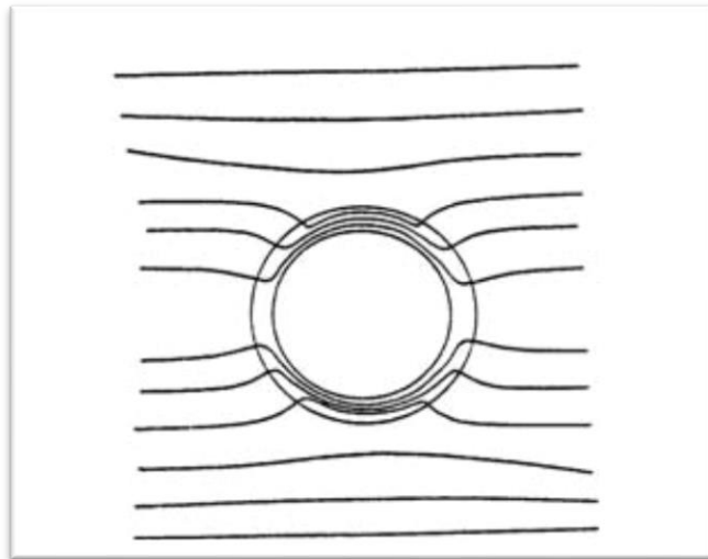
Figura 7: andamento qualitativo della deformazione delle linee di forza di un campo magnetico uniforme per effetto di un nucleo in materiale ferromagnetico
