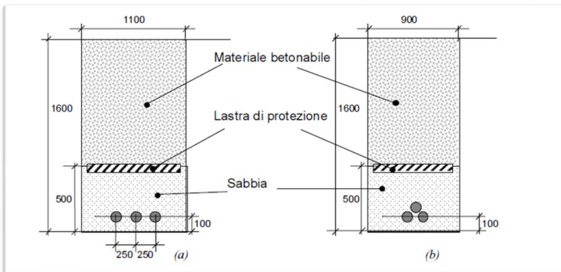
Figura 8: schermatura cavi elettrici interrati
