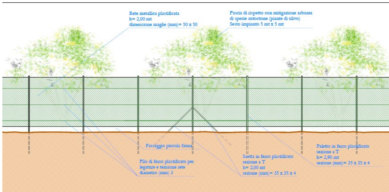
Figura 7 – Particolare recinzione perimetrale e opere di mitigazione (vista frontale)_scala 1:50
