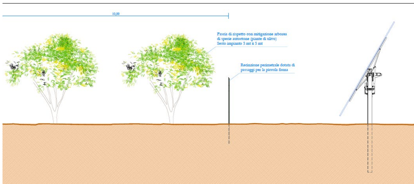
Figura 8 – Particolare recinzione perimetrale e opere di mitigazione (vista laterale) _scala 1:50
