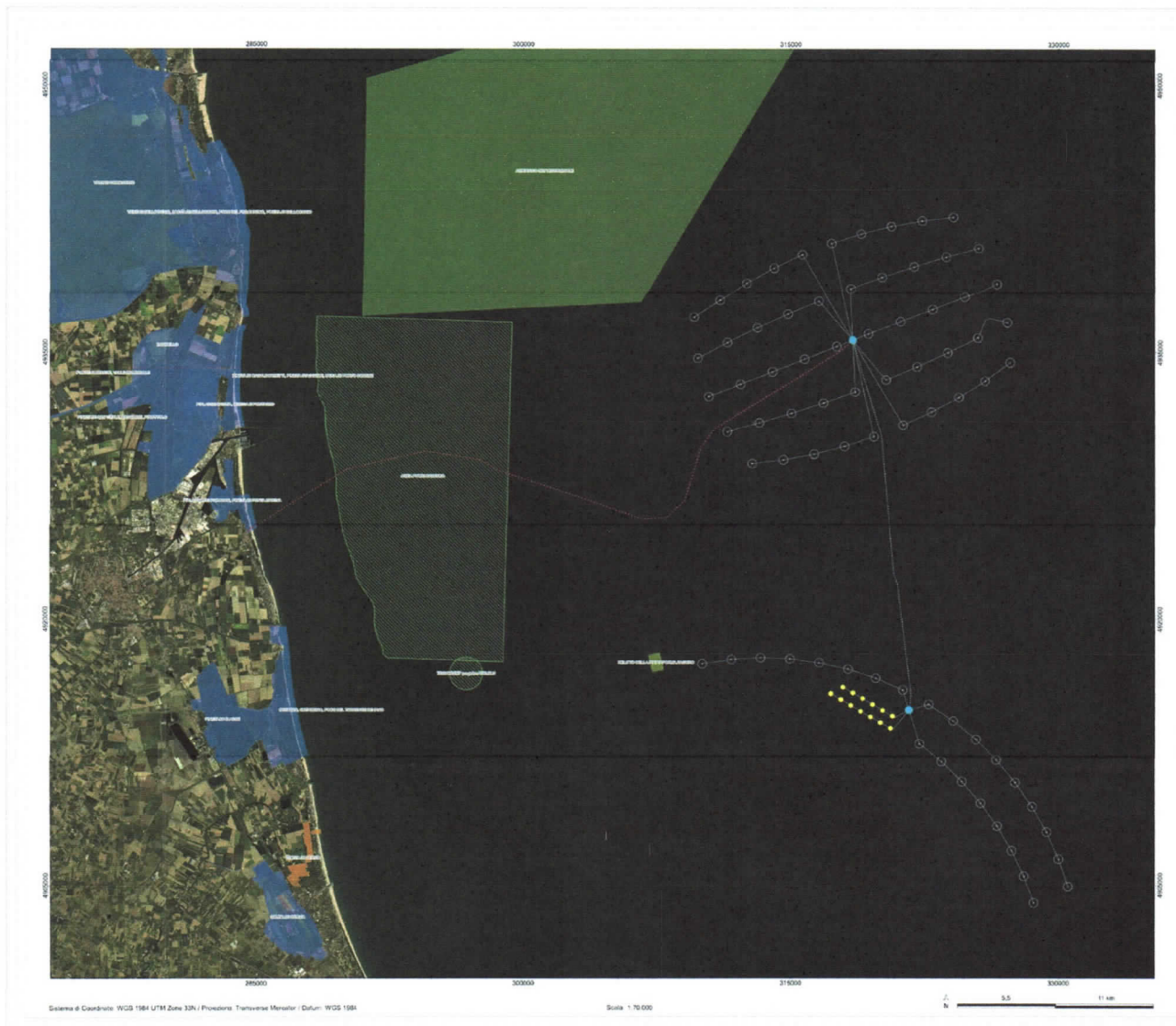
Tavola: AGNROM_EP-D_INQ-AMB-MARE - Inquadramento delle opere a mare su sintesi dei principali vincoli ambientali. I cerchi rossi evidenziano la vicinanza delle opere di progetto al SIC mare Adriatico Settentrionale, e alla ZSC Piattaforma Paguro. E' indicato inoltre l'areale dell'impianto fotovoltaico.
