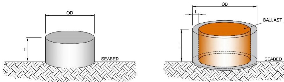
Figura 4-1: Schema Semplificato di Ancore a Gravità Piene (Sinistra) o Cave con Zavorra (Destra)
