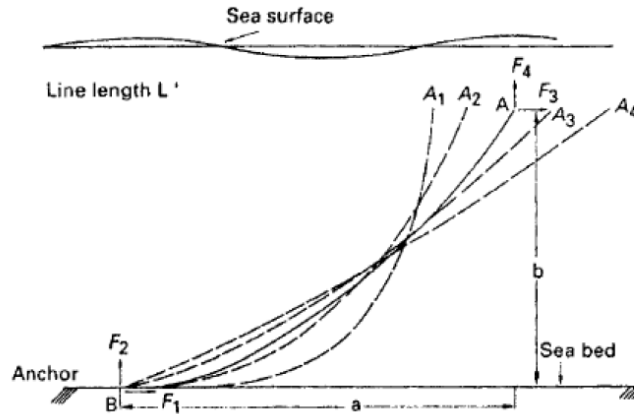
Figura 3-2: Sistema di Ormeggio con Catenaria [1]
