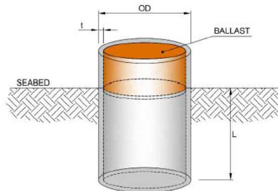
Figura 4-3: Schema Semplificato di Ancore Ibride
