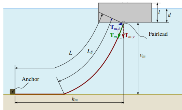
Figura 3-3: Catenaria
