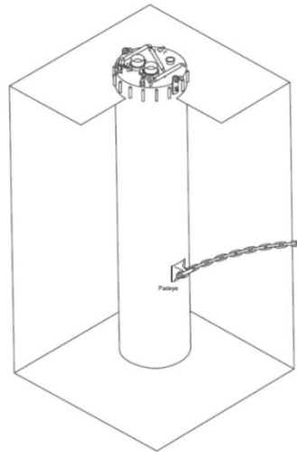
Figura 4-2: Tipica Connessione tra 'Suction Pile' e Linea di Ormeggio a Catenaria [8]
