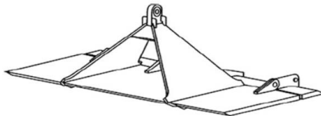
Figura 4-8: Esempio Schematico di Ancora a Piastra [4]
