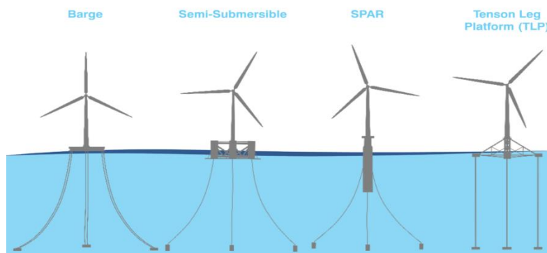
Figura 3-1: Esempi di Strutture Galleggianti per Parchi Eolici
