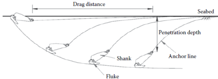
Figura 4-5: Schema di Installazione di Ancore a Trascinamento DEA [24]
