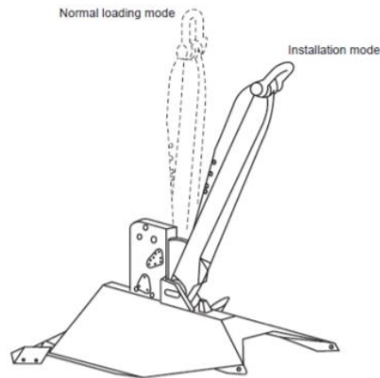
Figura 4-7: Variazione Angolo 'Shank-Fluke' Installazione/Esercizio per Ancora Bruce Dennla VLA [5]
