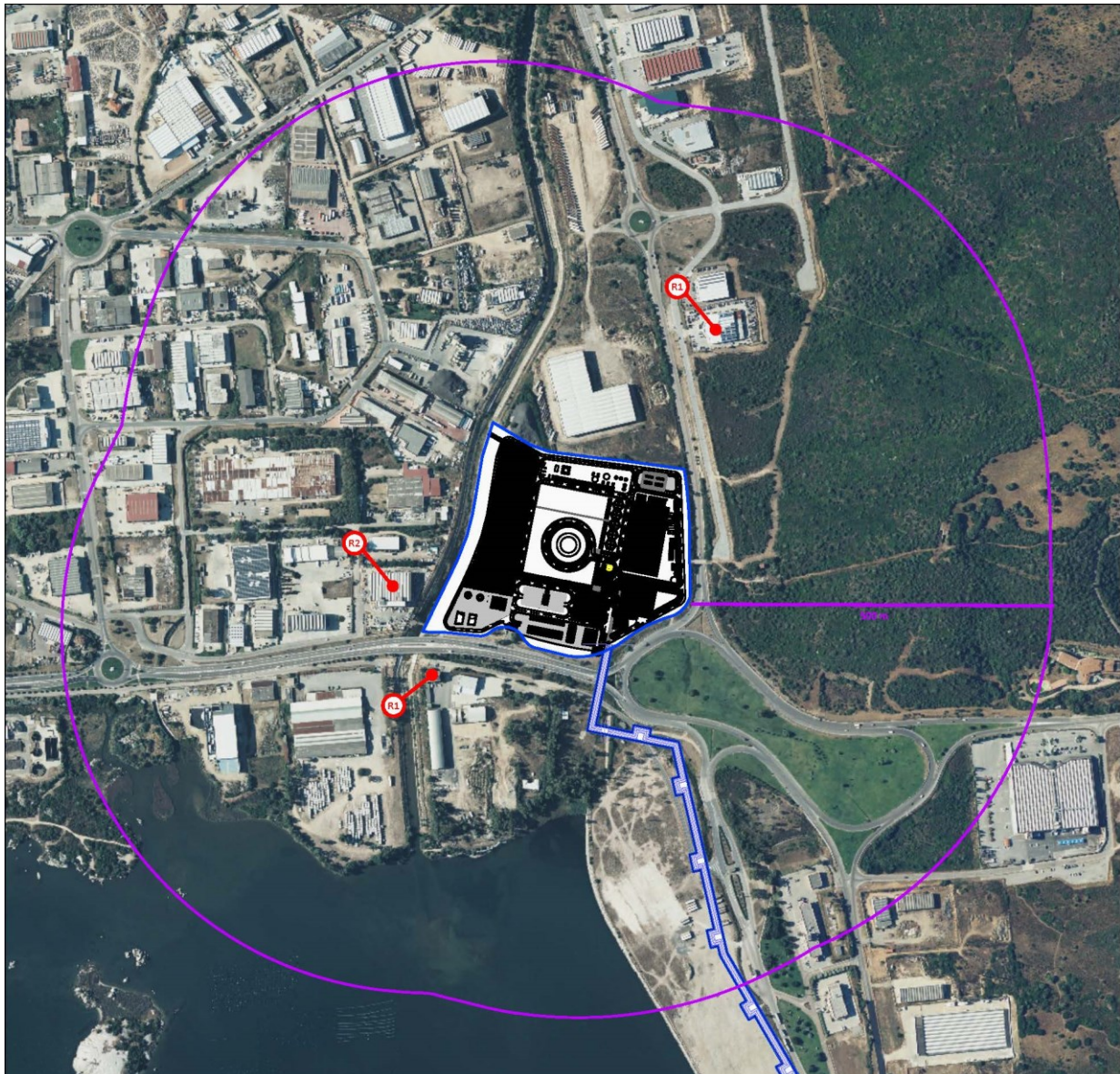
Figura 3 - Pianta del sito con i recettori individuati e involucro area di influenza pari a 500 m dal confine dello stabilimento
