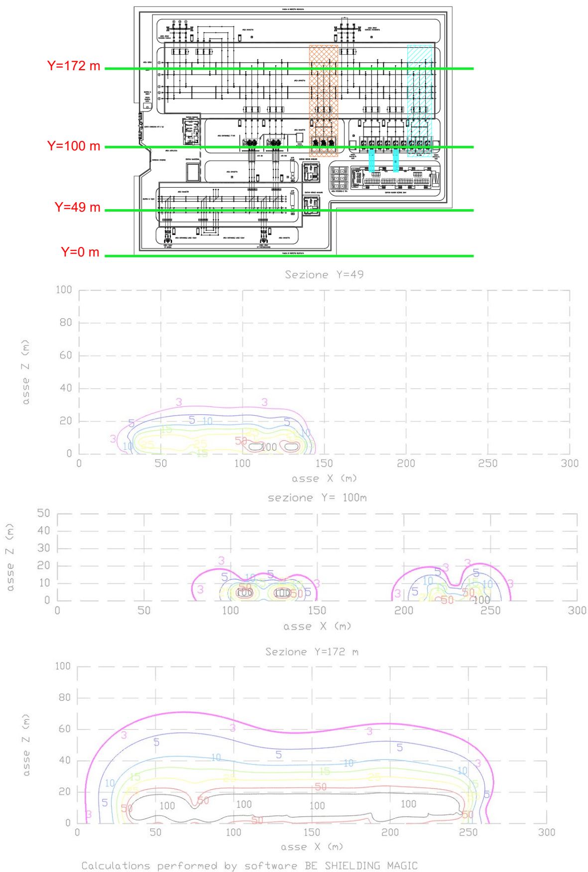
Figura 6 – Livelli di campo magnetico generato sul piano XZ in diversi punti della stazione
