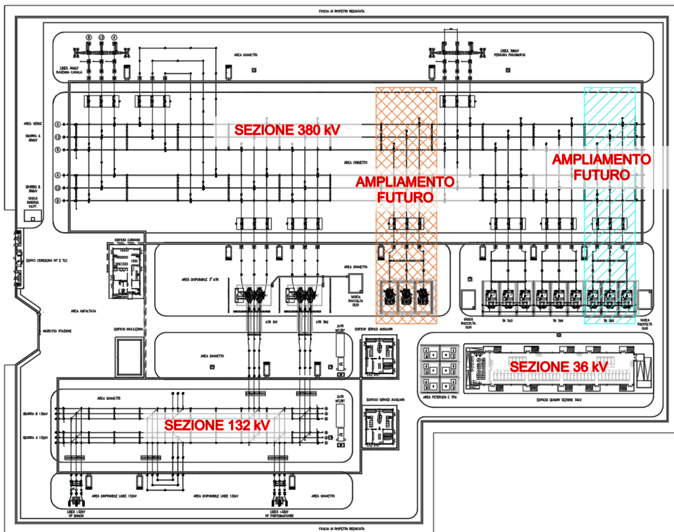
Figura 1: planimetria della stazione
