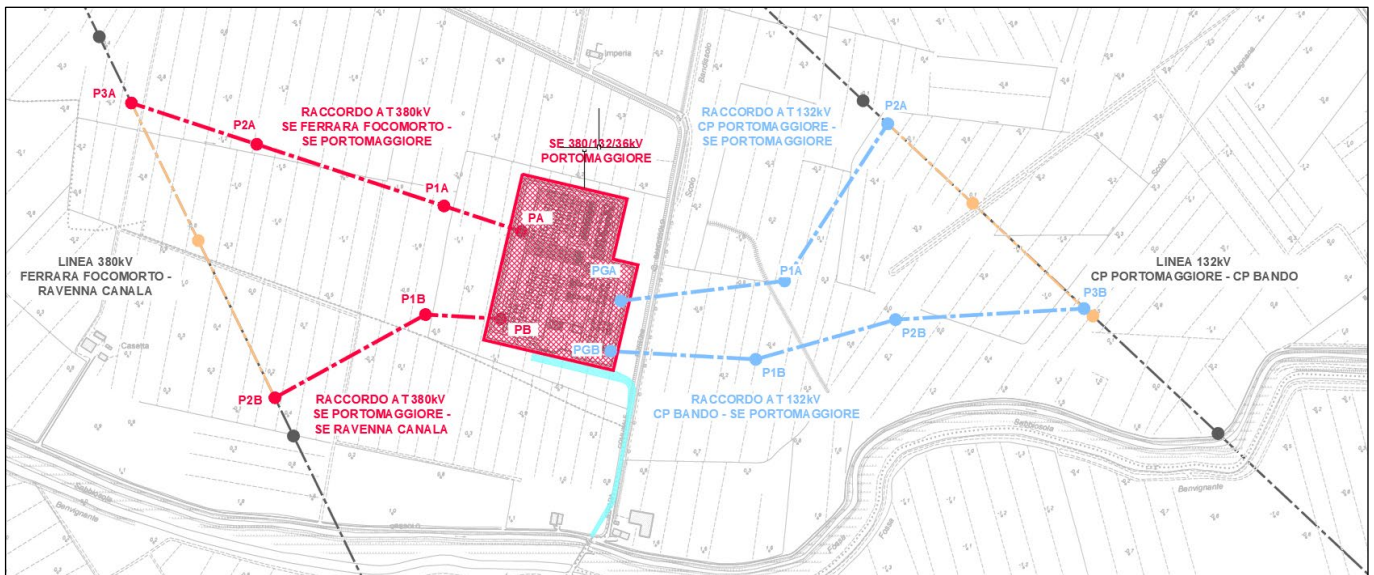
Figura 1: stralcio della planimetria con indicazione delle opere in progetto
