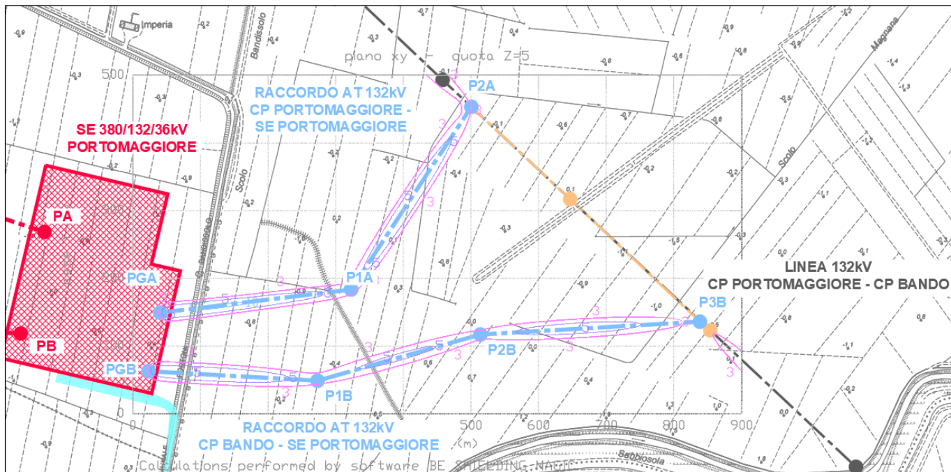
Figura 4 – Livelli di campo magnetico generato dai raccordi a 132 kV a 5 mslm
