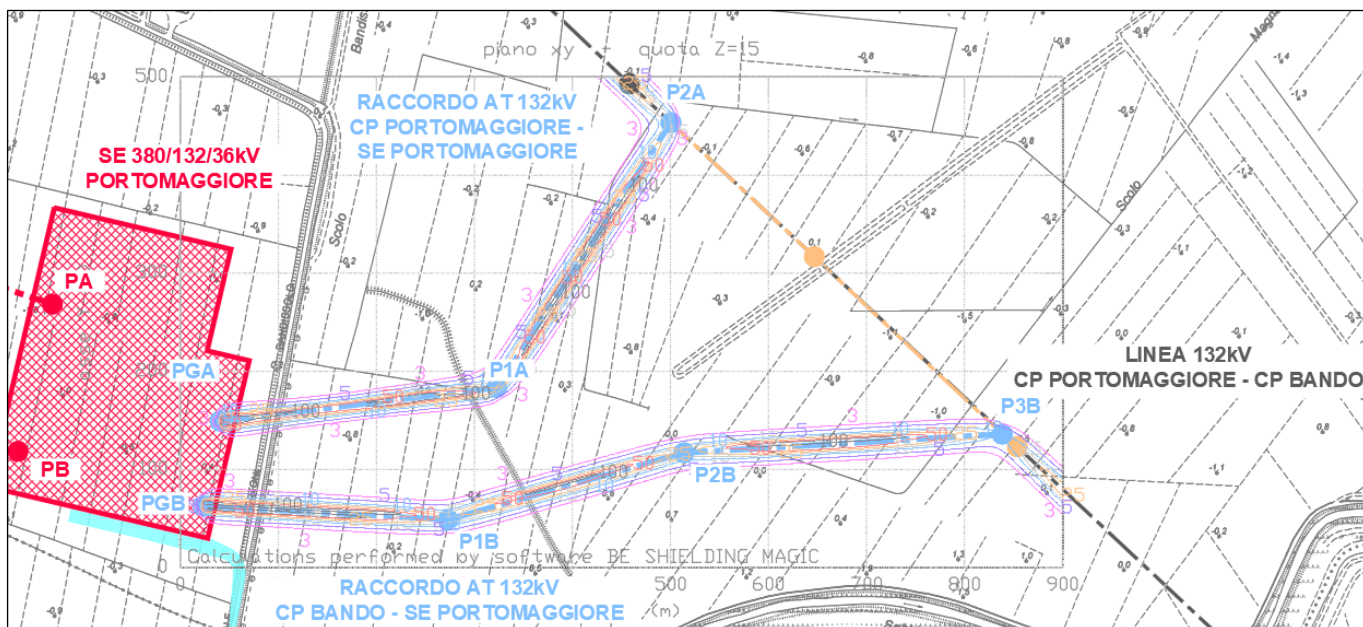
Figura 5 – Livelli di campo magnetico generato dai raccordi a 132 kV a 15 mslm
