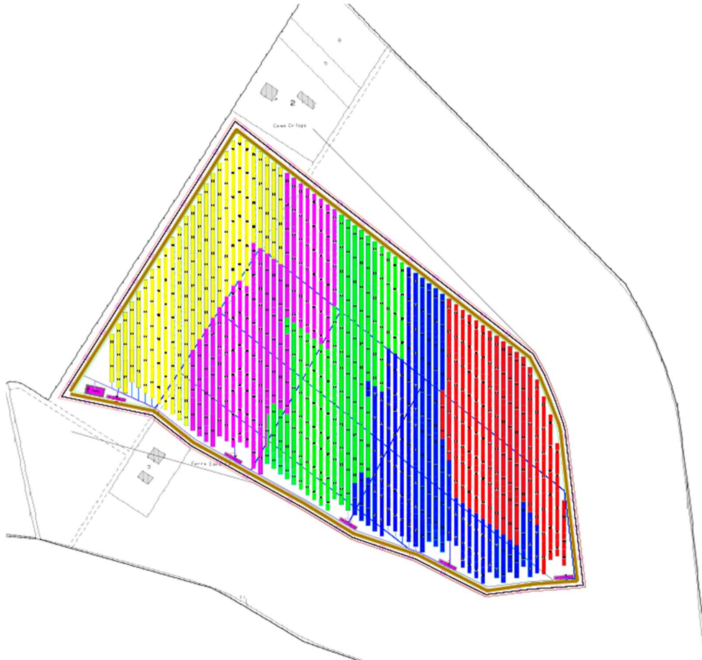
Figura 3: Layout preliminare di impianto
