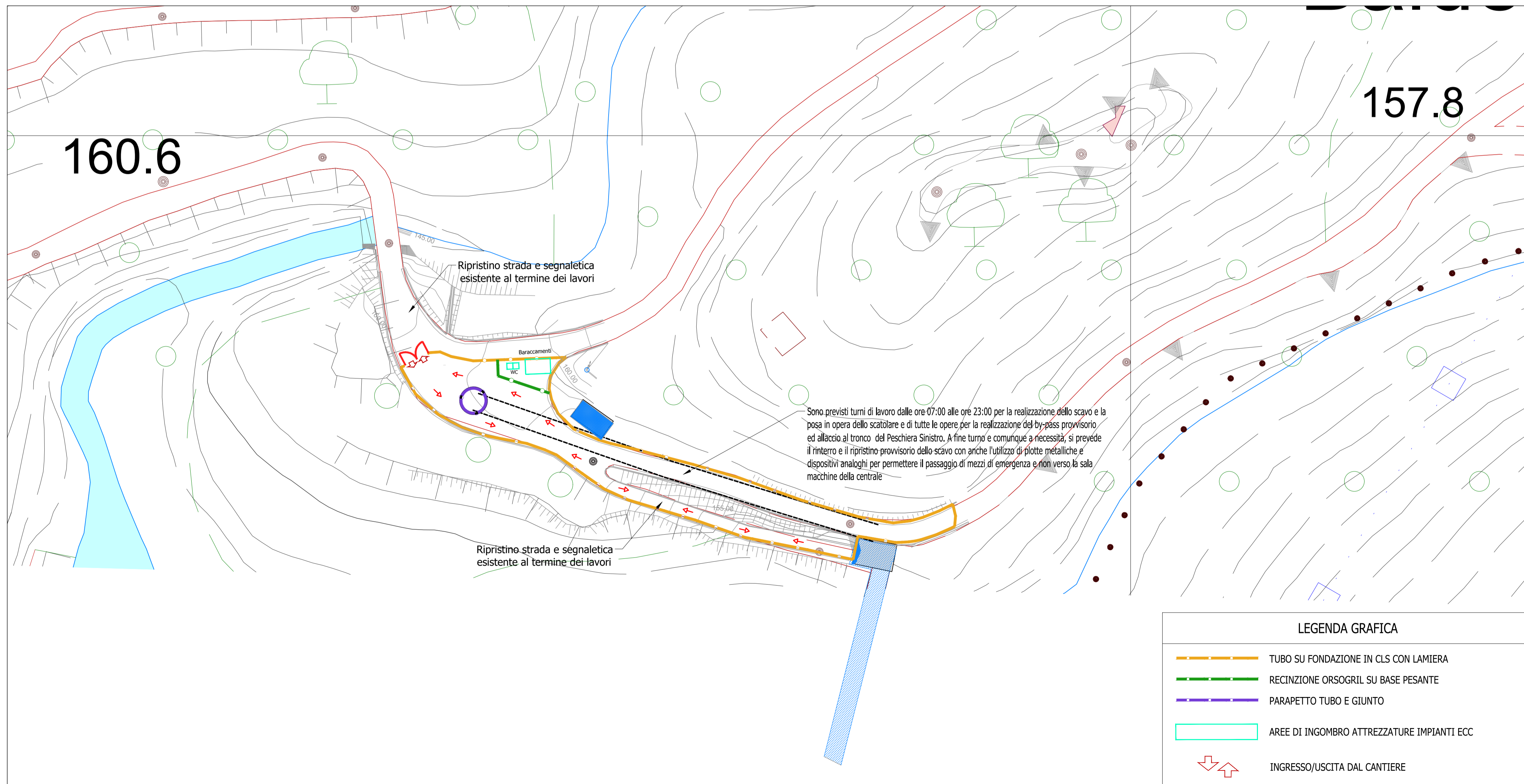
PLANIMETRIA DI CANTIERE - SCALA 1:500
