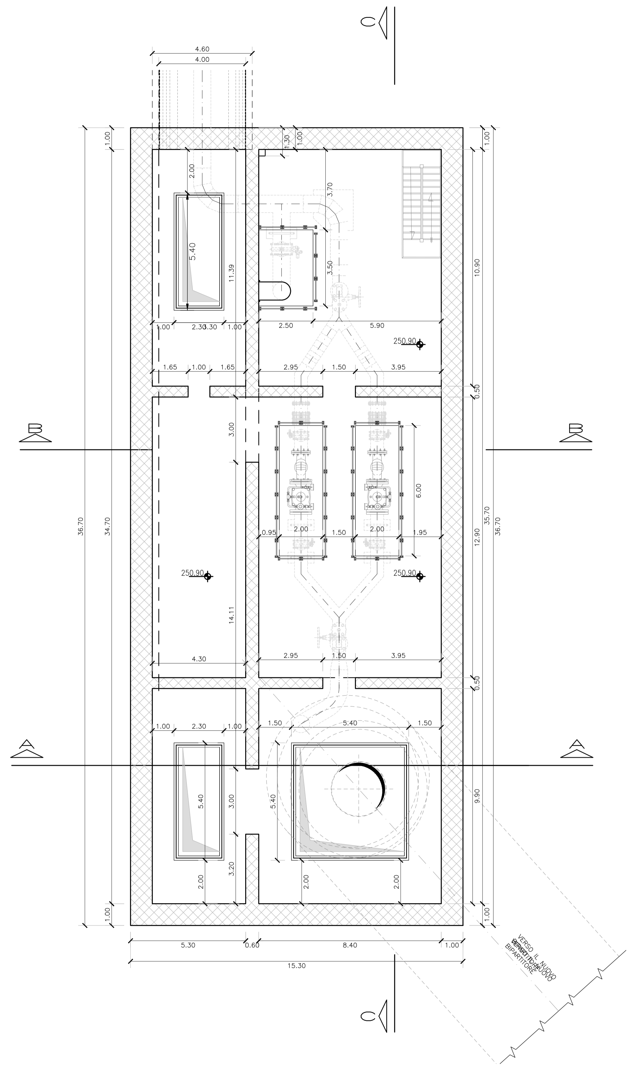
PIANTA E-E - SCALA 1:100
