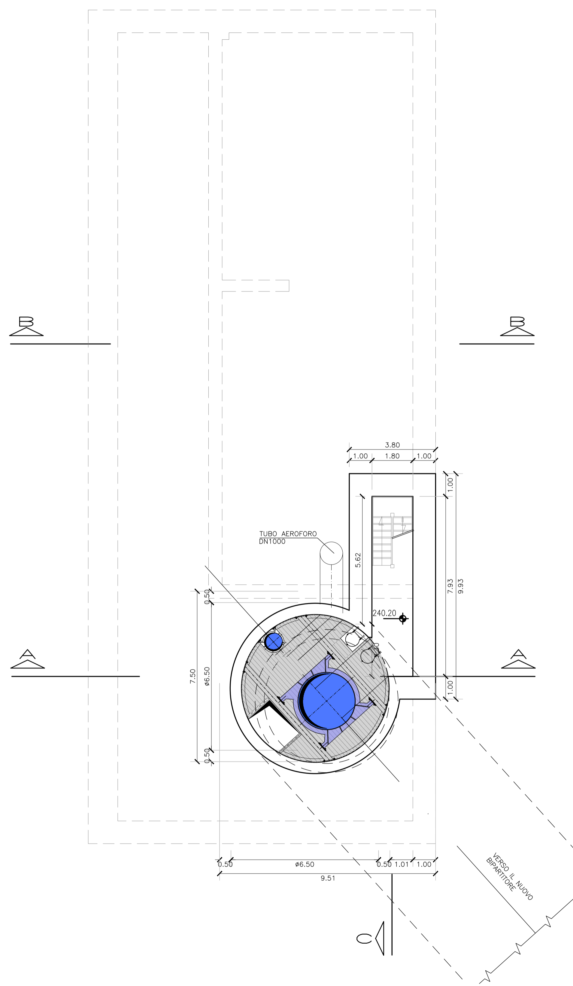
PIANTA D-D - SCALA 1:100
