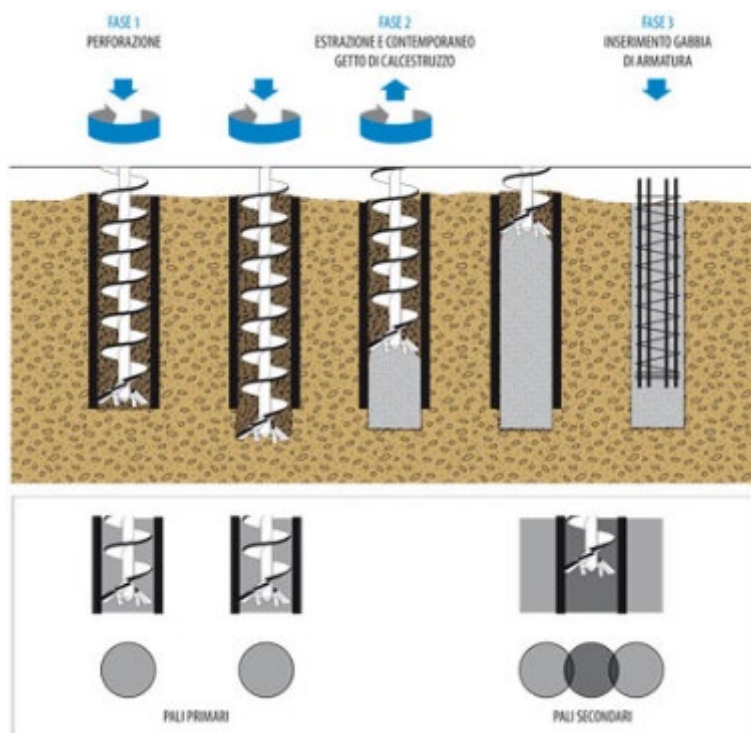
Figura 7.2 - Schema esecutivo pali secanti CSP
