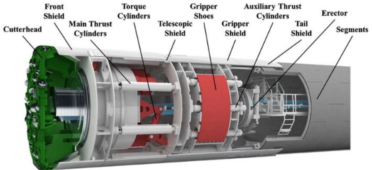
Caratteristiche della ROCK-TBM DN7500
