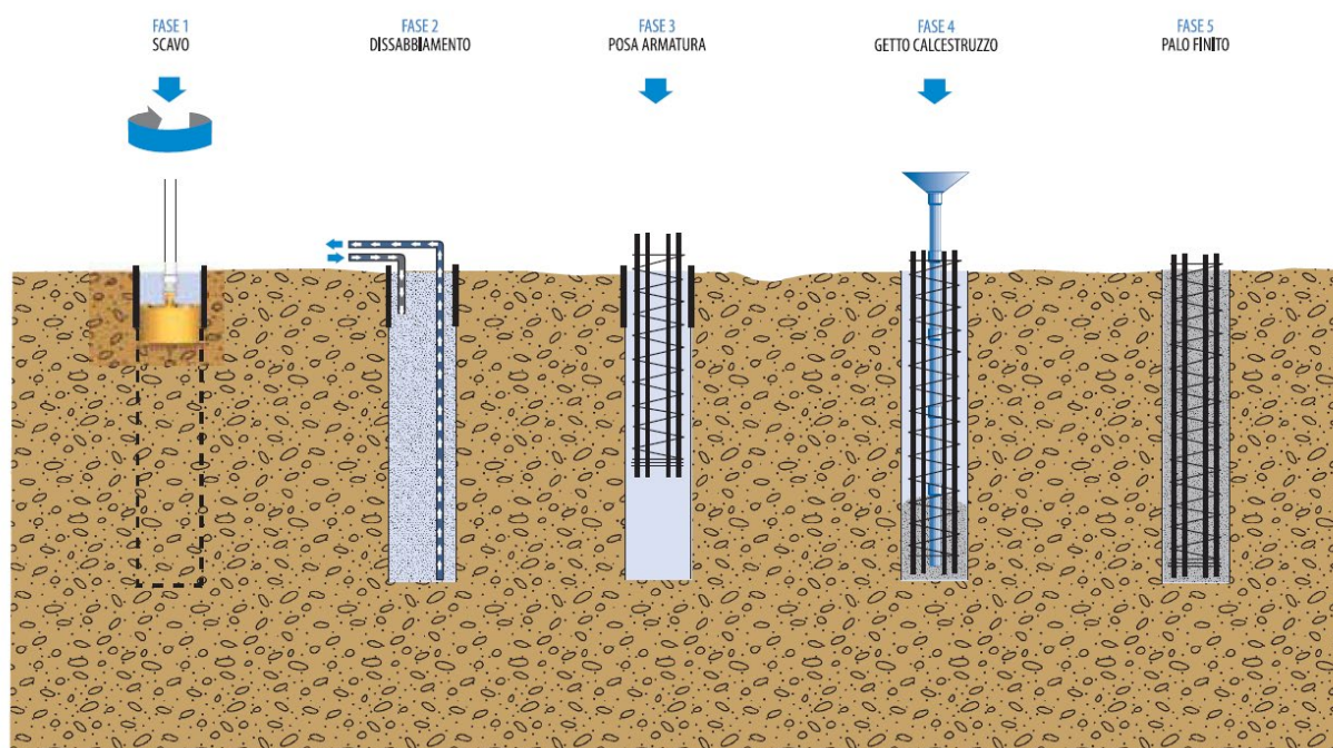
Figura 7.1 - Schema esecutivo pali trivellati classici
