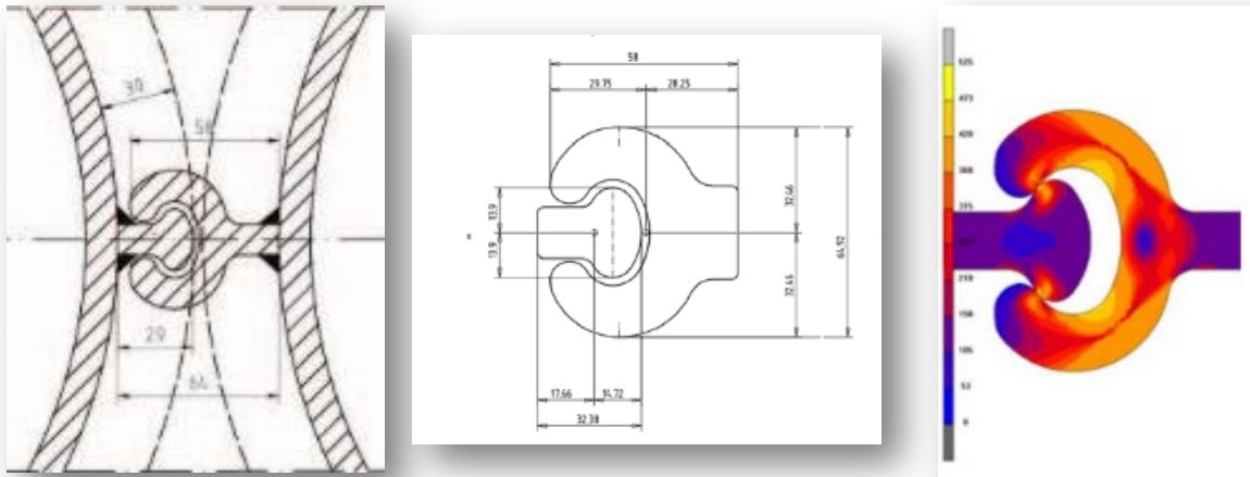
Figura 7.5 - Gargame ad omega
