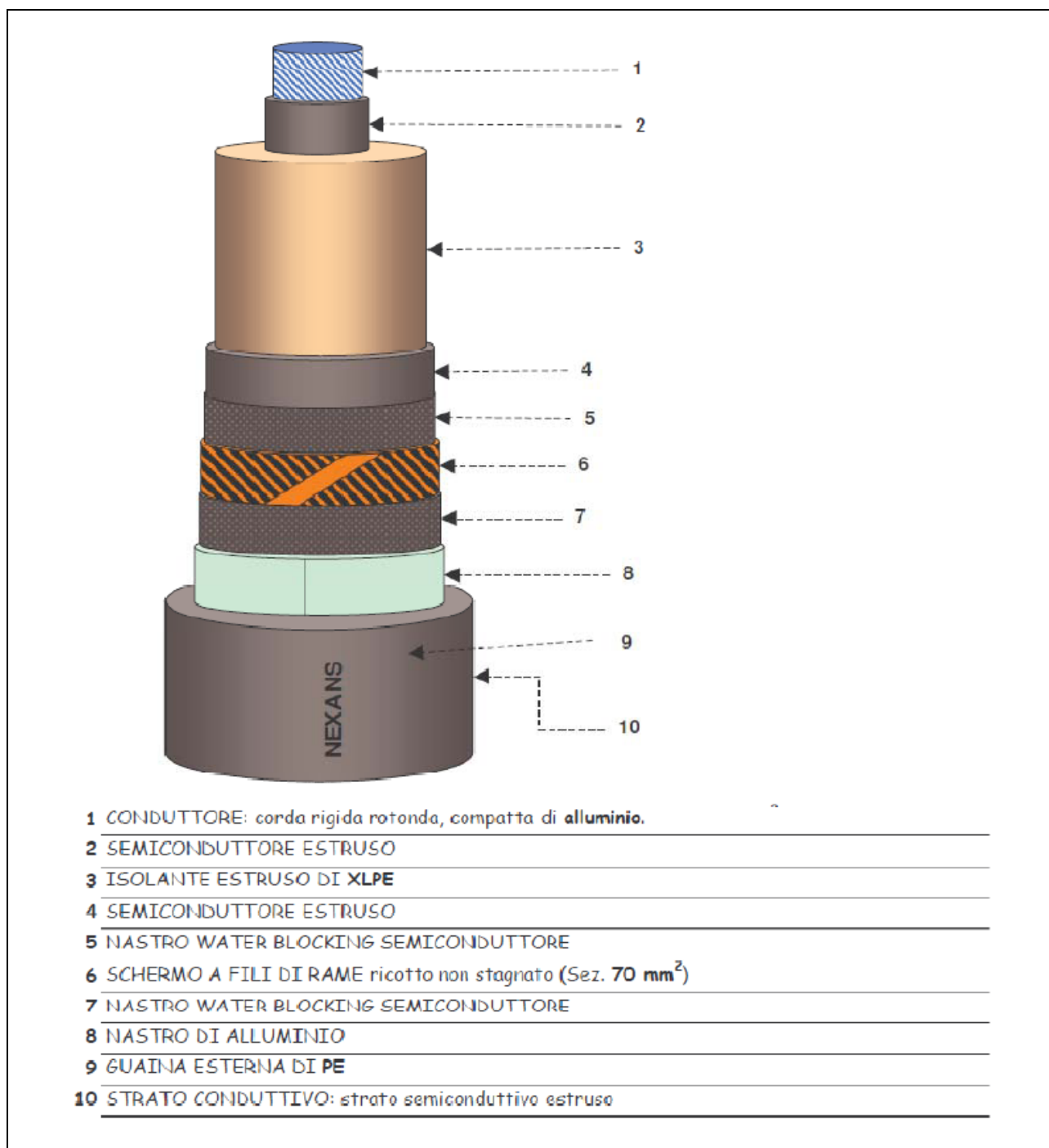
Schema tipico del cavo
