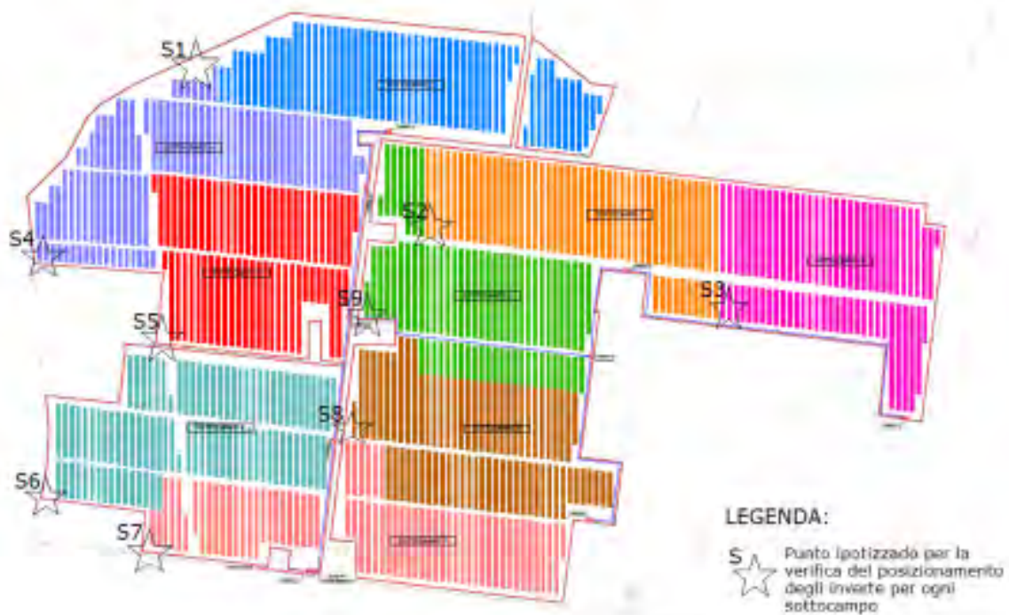
Figura 68 Planimetria con individuazione degli inverter ai fini del calcolo
