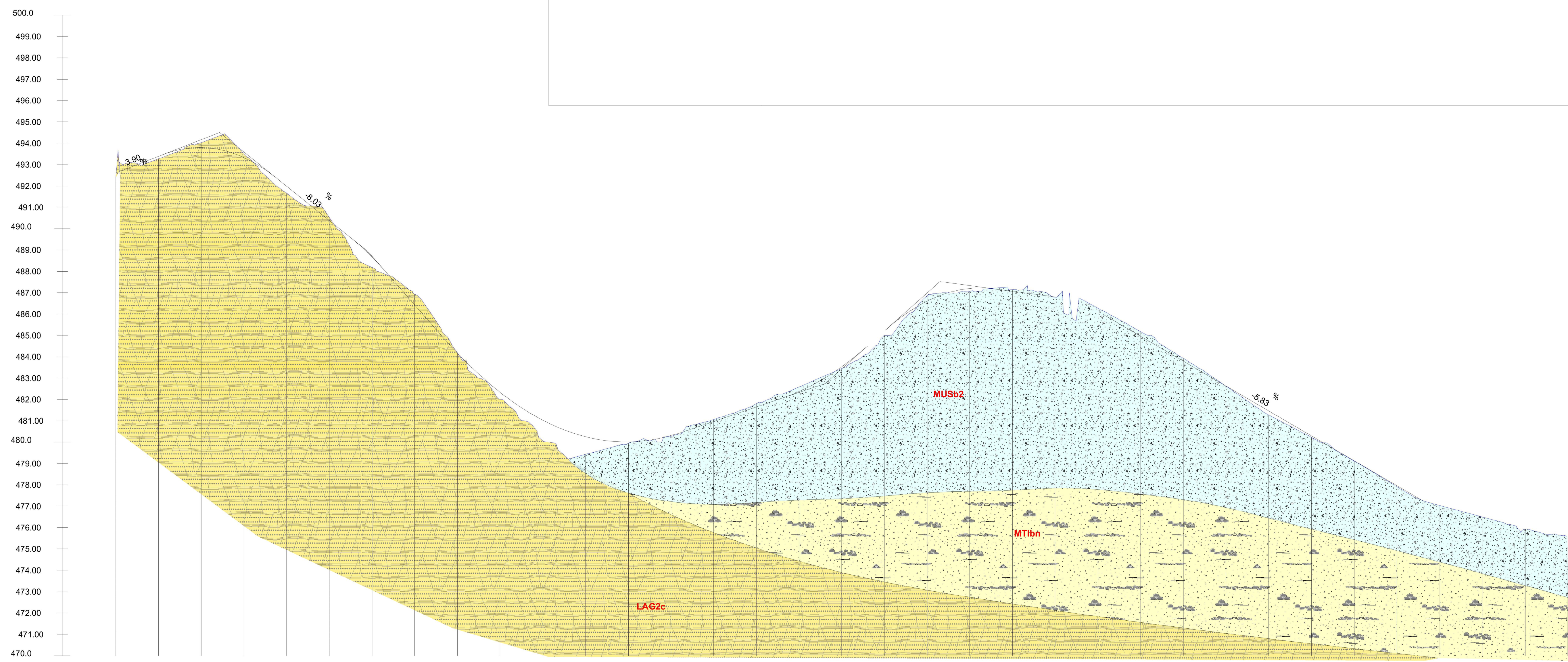
Profilo: VS 08-Profilo Scala: 1:1000 Q.Ref.: 470.00
