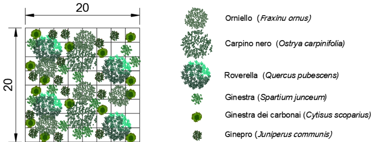
Figura 4-9 Sesto di impianto previsto per il rimboschimento con specie arboree/arbustive autoctone
