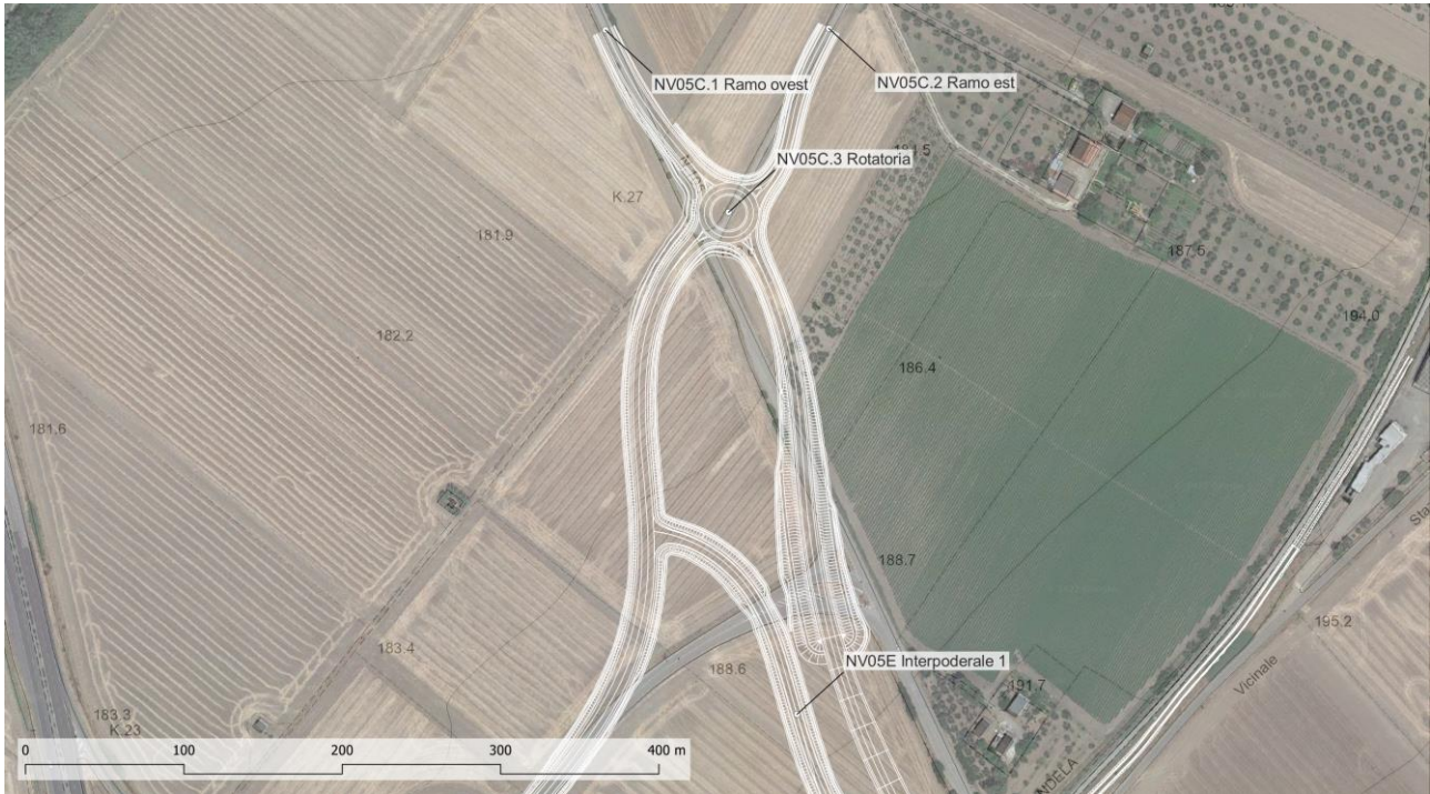
FIGURE 2 NV05 INQUADRAMENTO DELLE OPERE IN PROGETTO, TRATTO NORD
