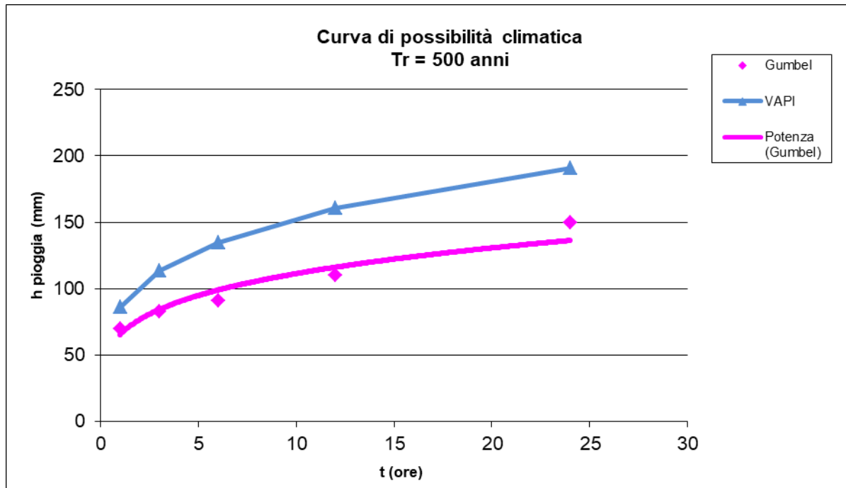
Figura 18: Curva di possibilità climatica con tempo di ritorno pari a 500 anni.
