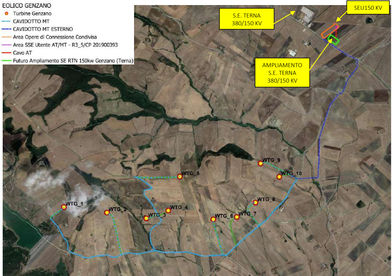
Figura 4: Layout di progetto su ortofoto.
