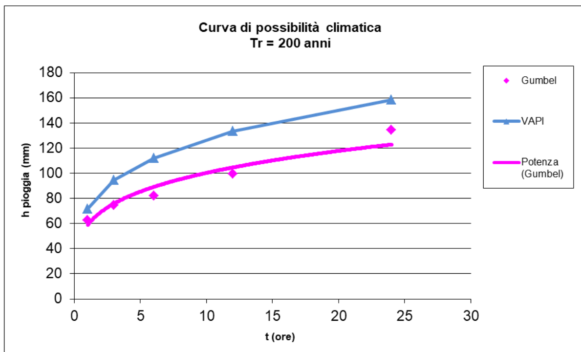
Figura 17: Curva di possibilità climatica con tempo di ritorno pari a 200 anni.
