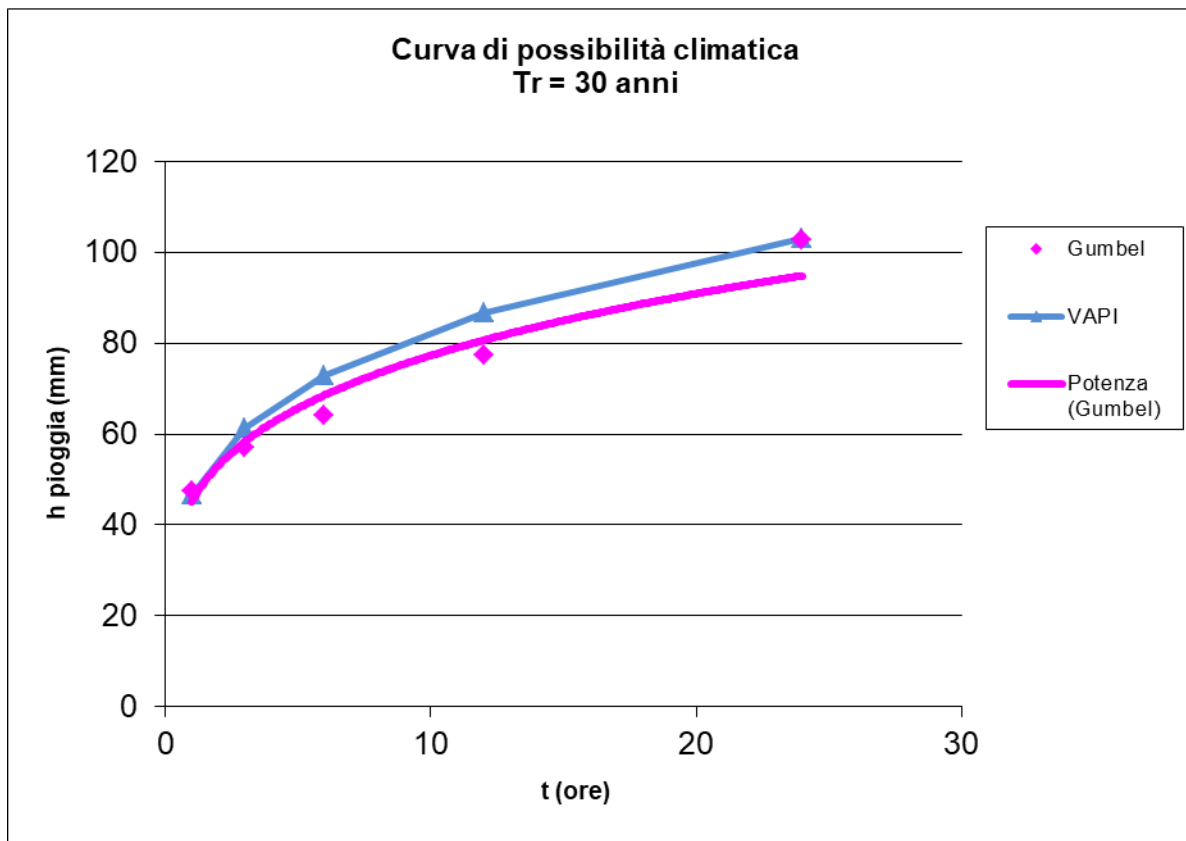
Figura 16: Curva di possibilità climatica con tempo di ritorno pari a 30 anni.
