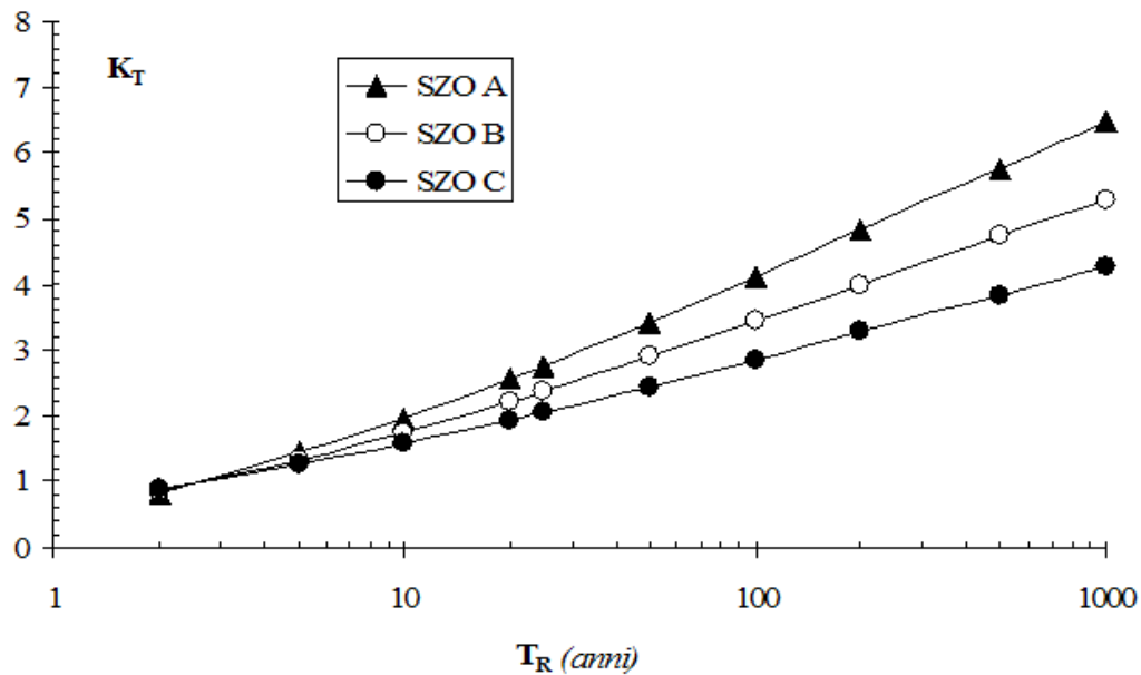
Figura 20: Andamento del fattore probabilistico di crescita delle piene.
