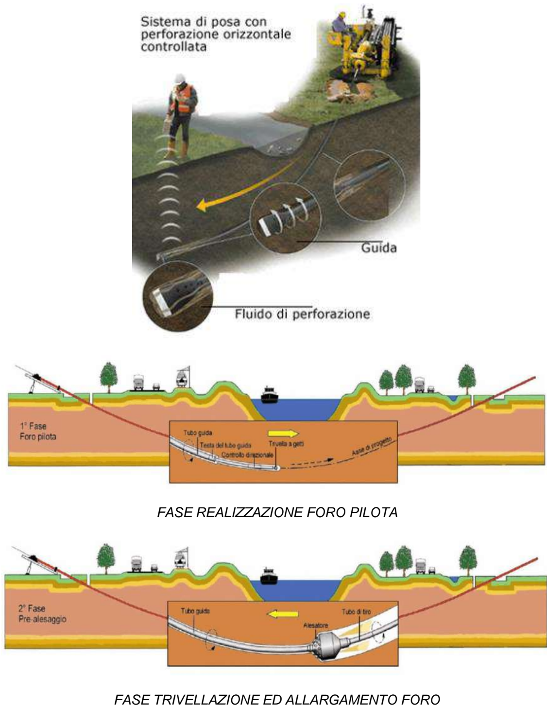
Figura 6: Sistema di trivellazione orizzontale controllata (TOC).
