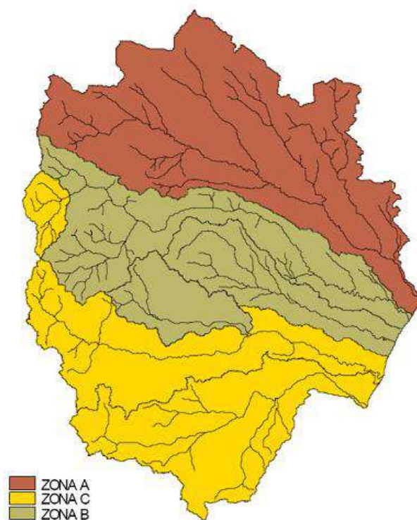
Figura 19: Sottozone omogenee al II livello di regionalizzazione delle piene.
