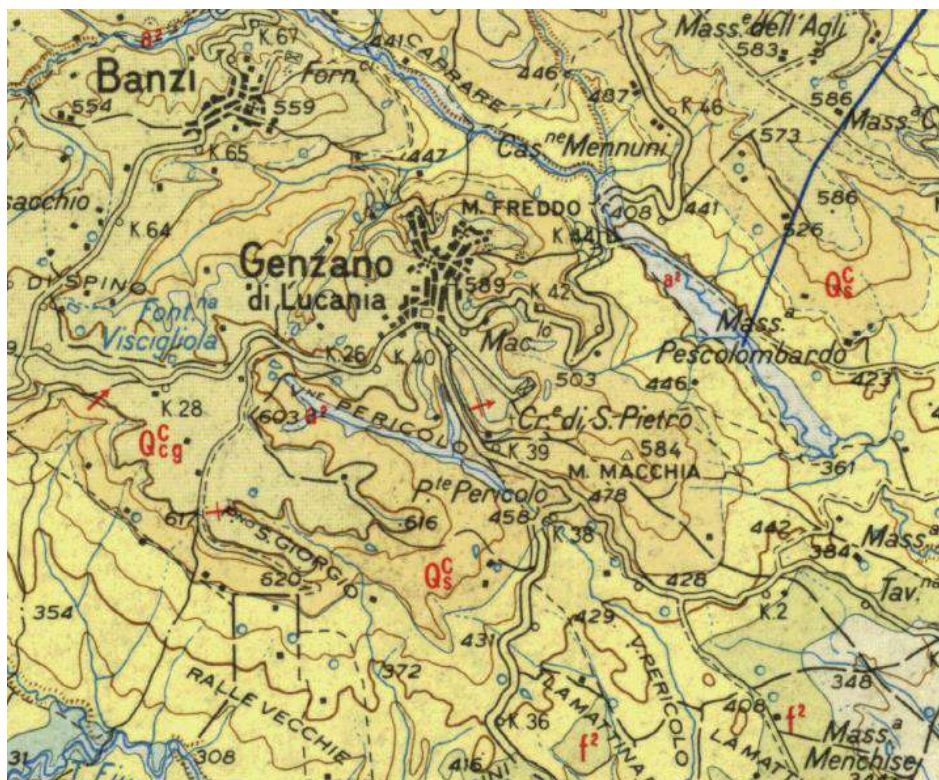
Figura 8: Stralci della carta geologica d'Italia (F.188, scala 1:100.000).
