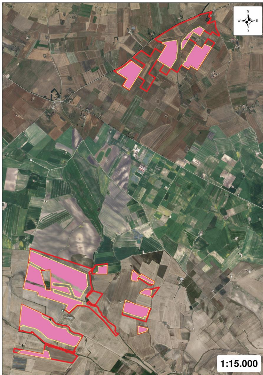
Figura 3 – Area di pertinenza del progetto con indicazione dell'ubicazione dei pannelli fotovoltaici e della recinzione perimetrale.
