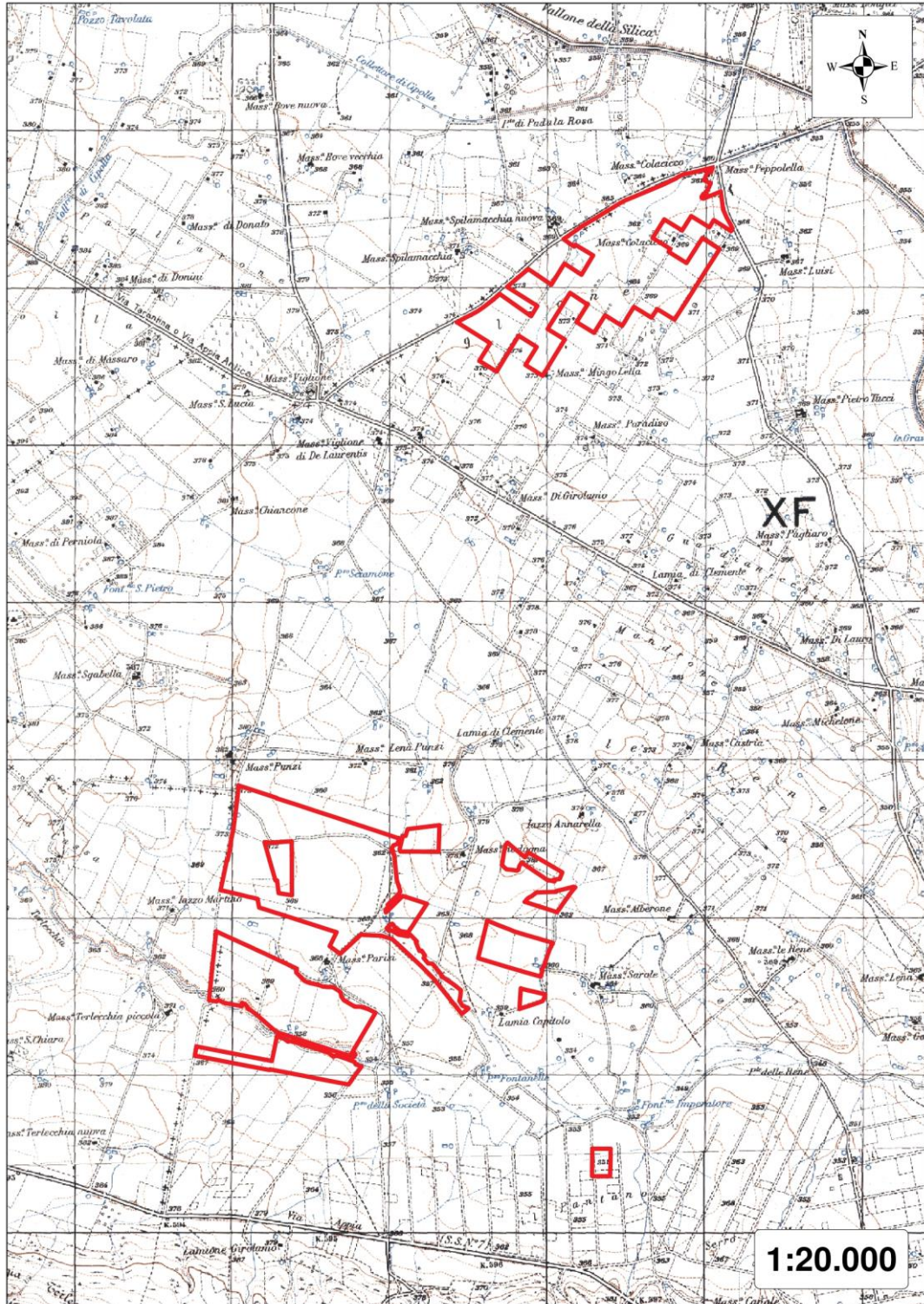
Figura 2 – Stralcio carta dell'I.G.M. con indicazione dell'area d'intervento
