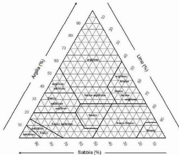
Figura 3. – Classificazione Tessitura del terreno USDA.
