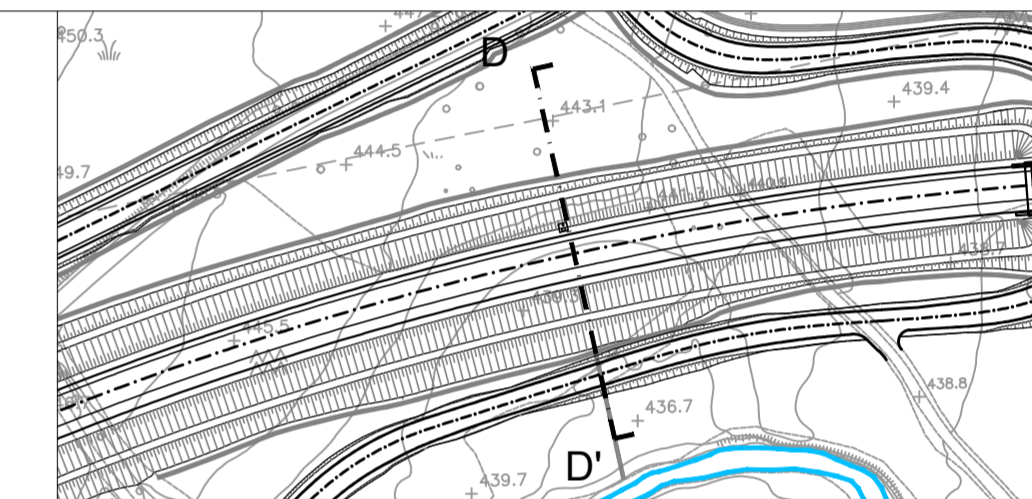
Pianta sezione DD' scala 1:2000
