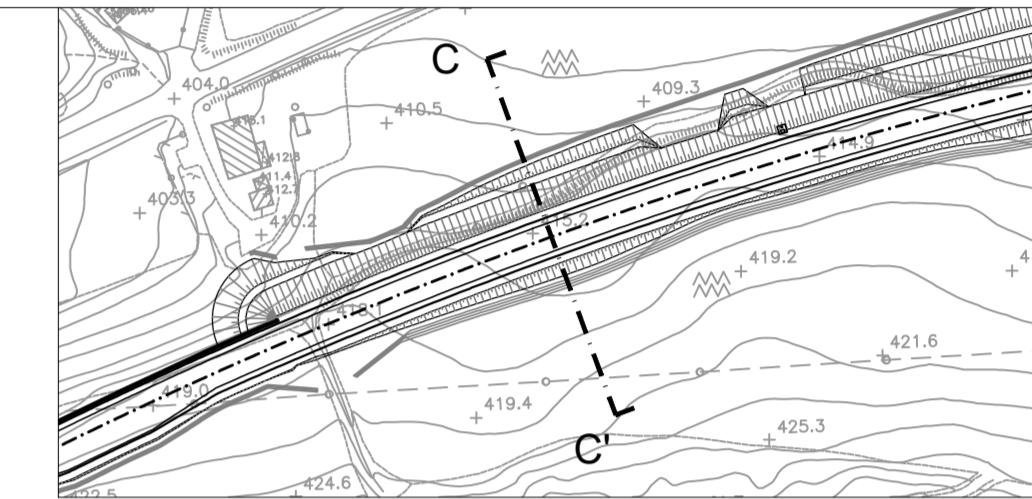
Pianta sezione CC' scala 1:2000
