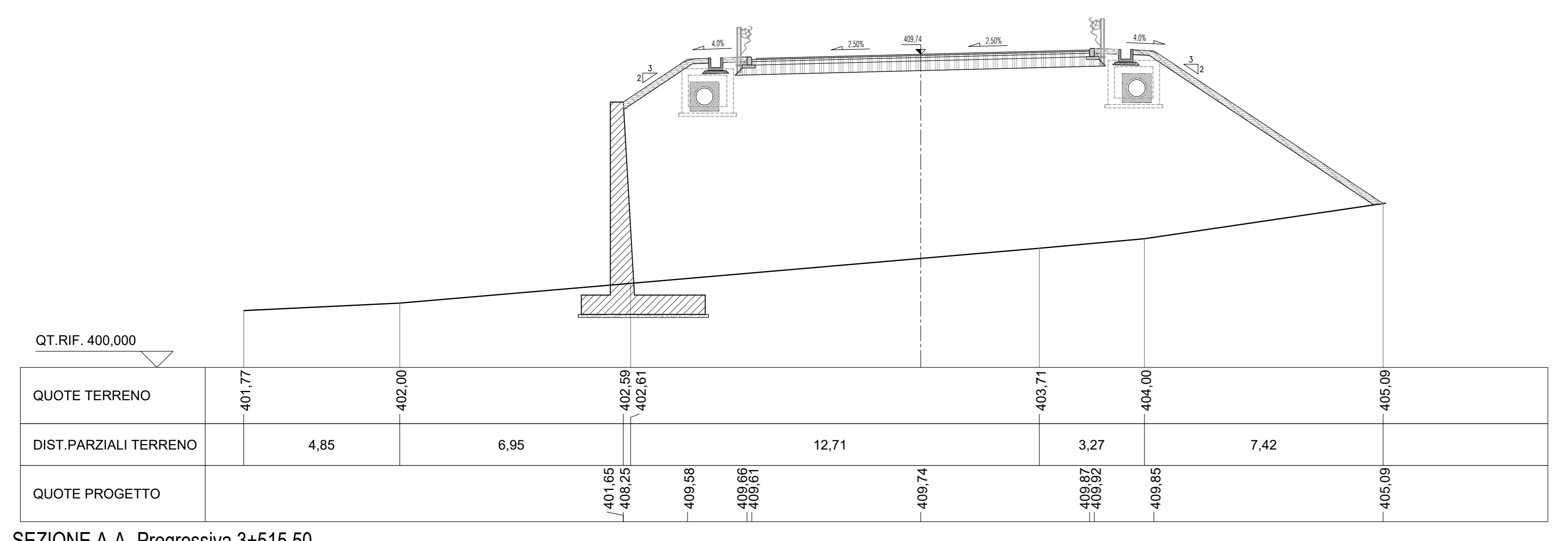
SEZIONE A-A-Progressiva 3+515.50 1:100
