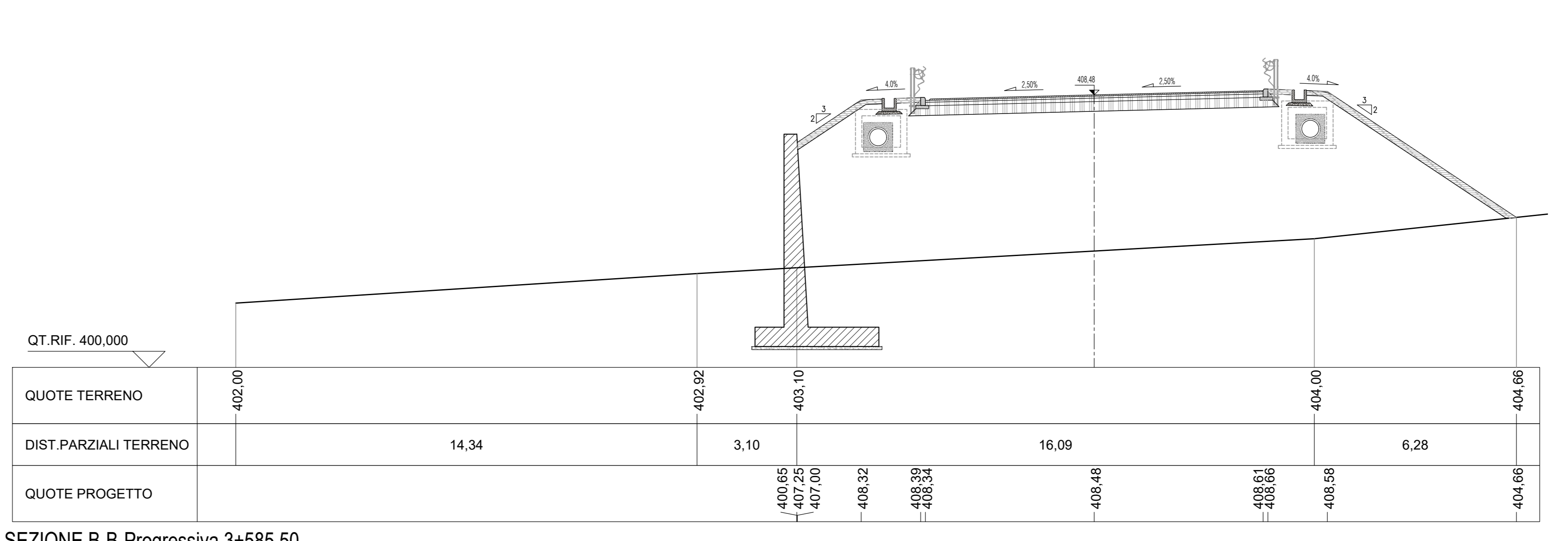
SEZIONE B-B-Progressiva 3+585.50 1:100
