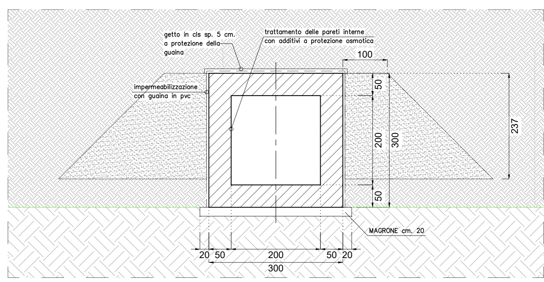
SEZIONE B-B 1:50
