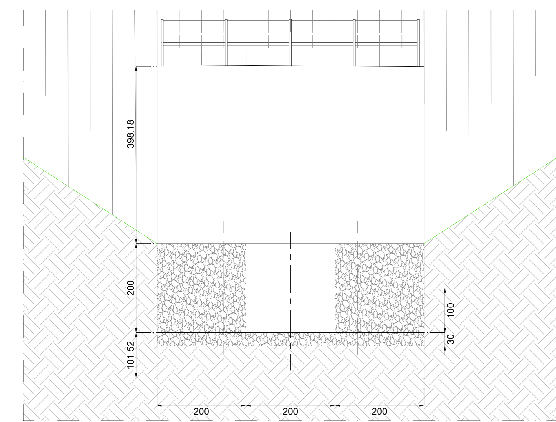
SEZIONE A-A 1:50
