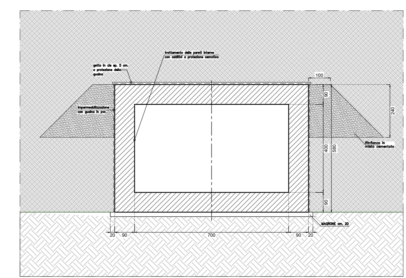
SEZIONE B-B 1:100
