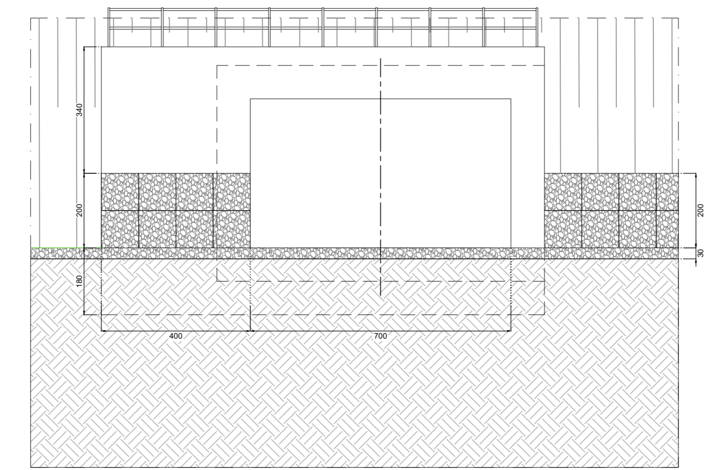
SEZIONE A-A 1:100
