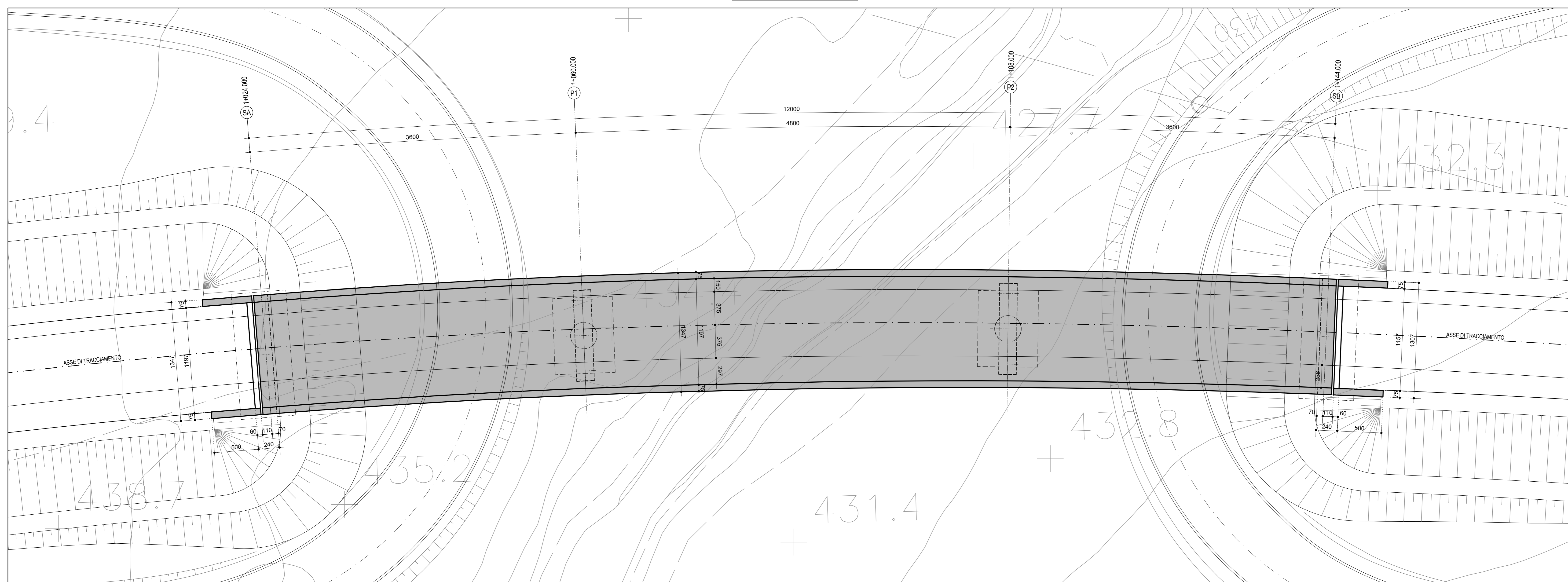
PIANTA IMPALCATO 1:200
