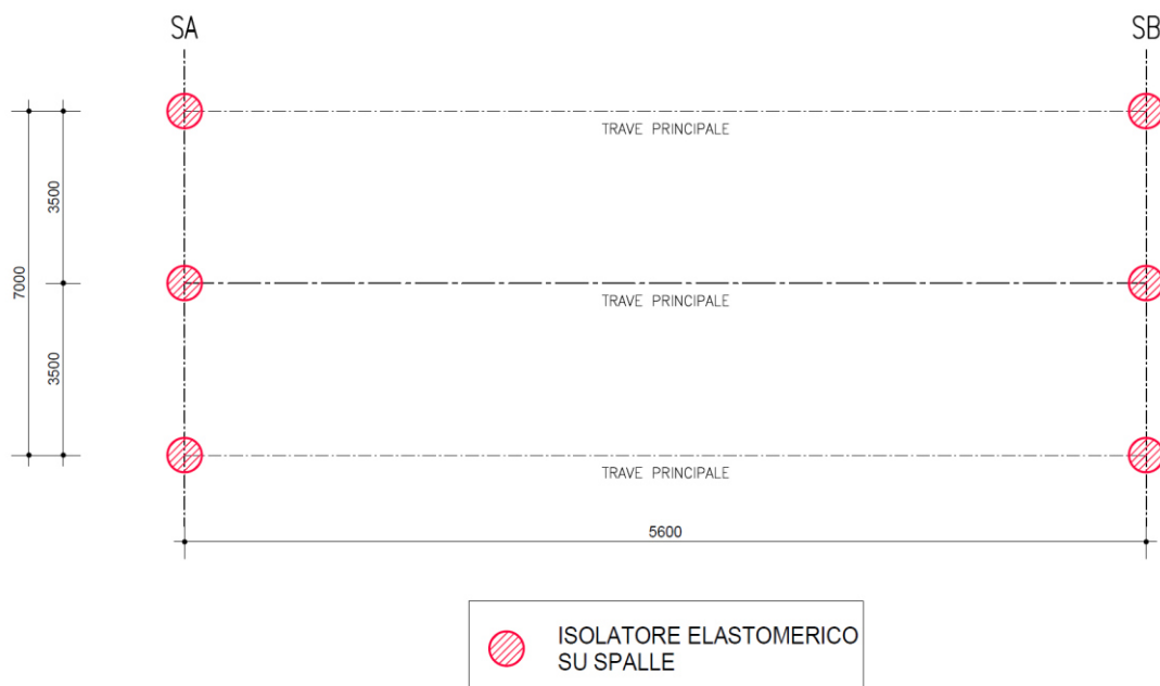
Figura 1- Schema appoggi
