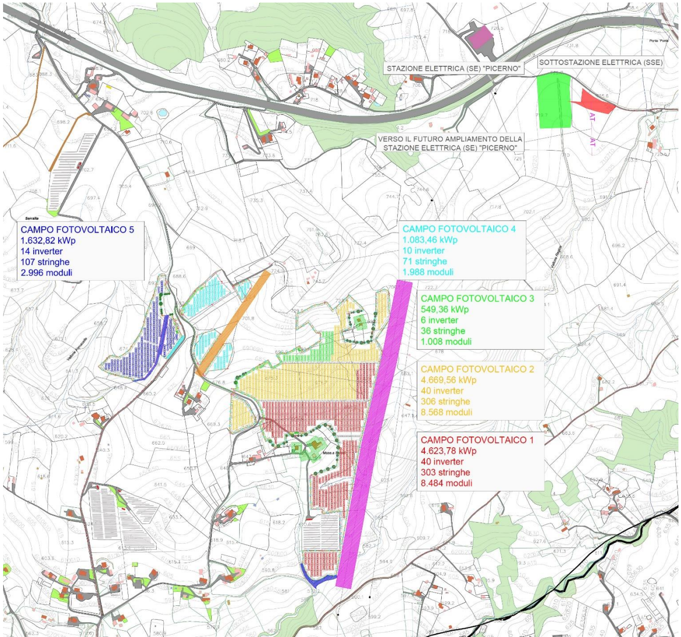
Schema di configurazione dei Campi Fotovoltaici e delle Opere di Rete previste da Progetto
