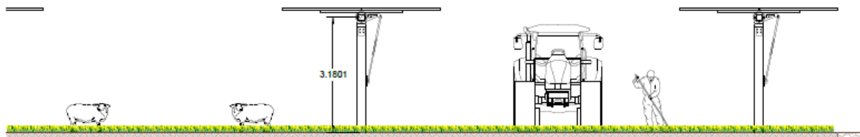
Figura 6 | Sezione trasversale tipologica interfilare delle strutture di sostegno dei moduli
