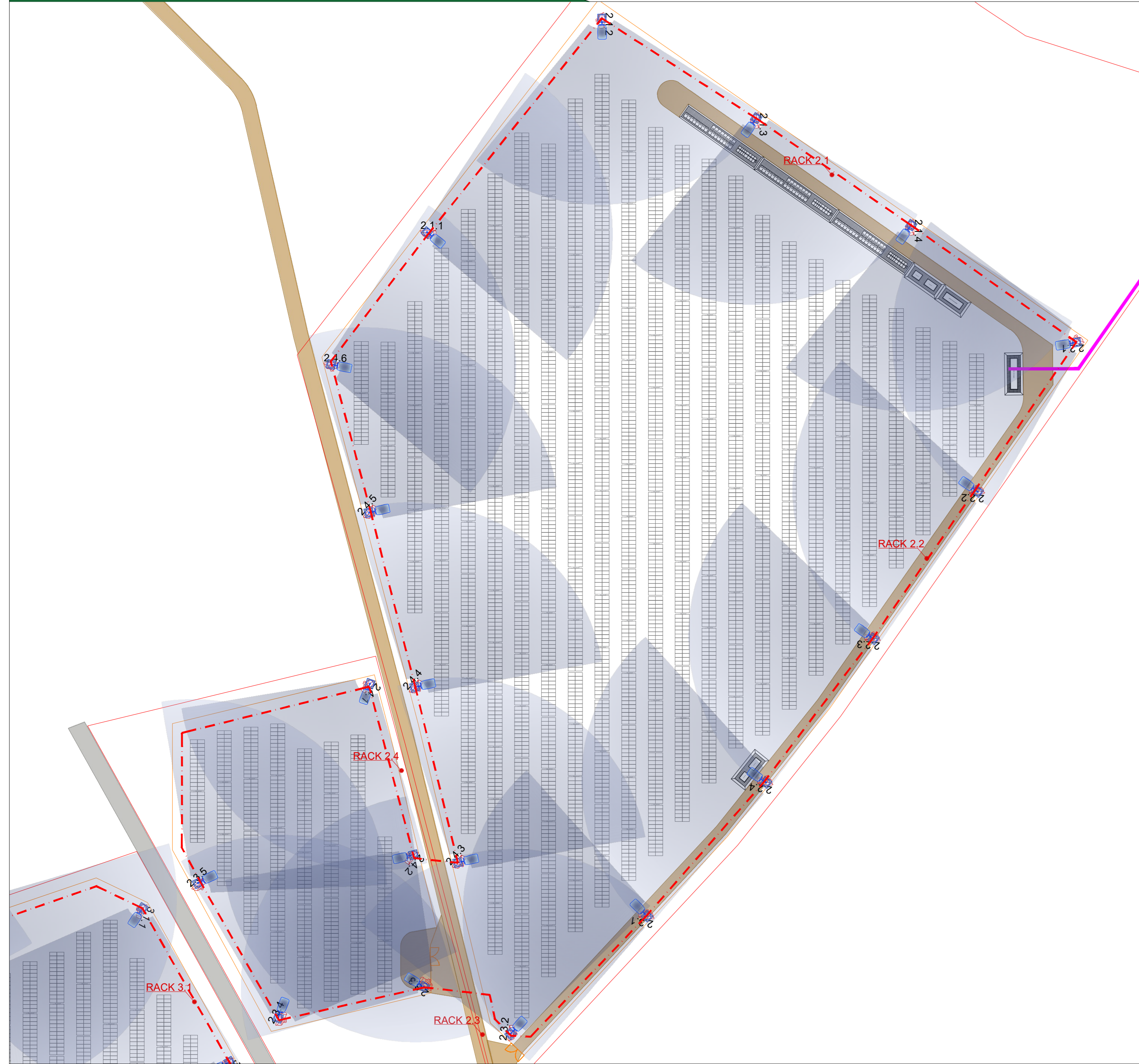
Layout impianto fotovoltaico - SISTEMA 2 - Scala 1:1000
