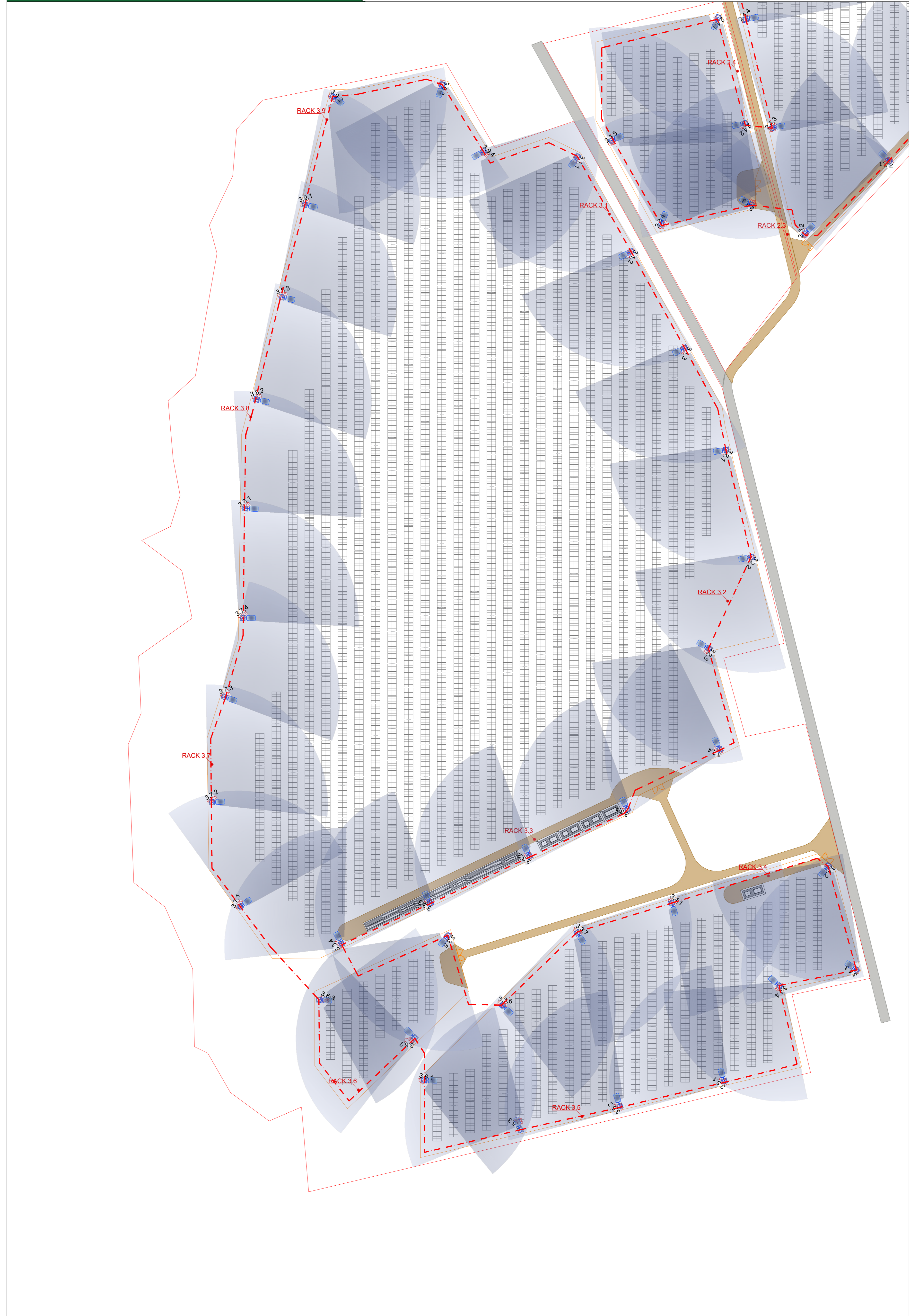
Layout impianto fotovoltaico - SISTEMA 3 - Scala 1:1000
