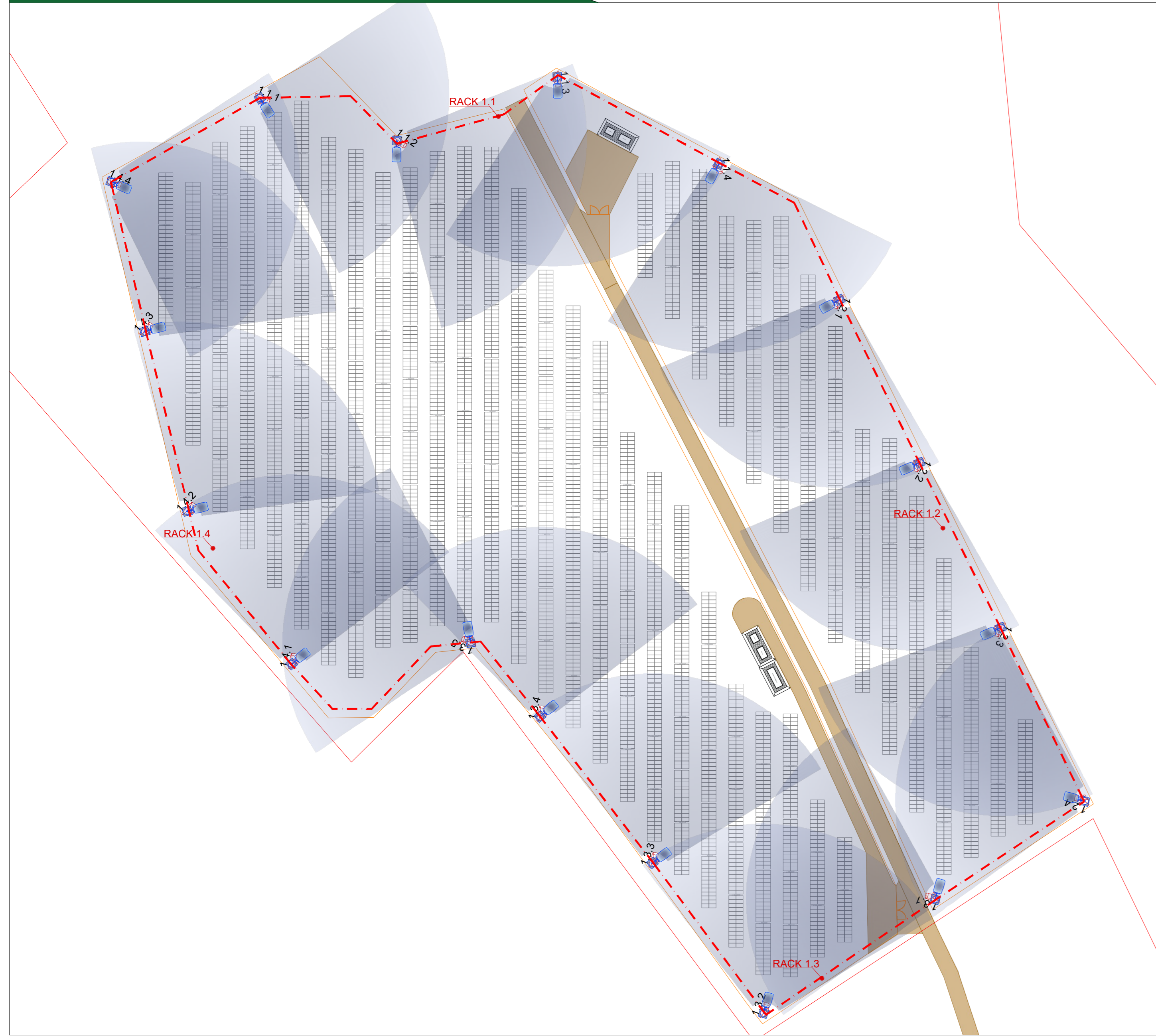
Layout impianto fotovoltaico - SISTEMA 2 - Scala 1:1000
